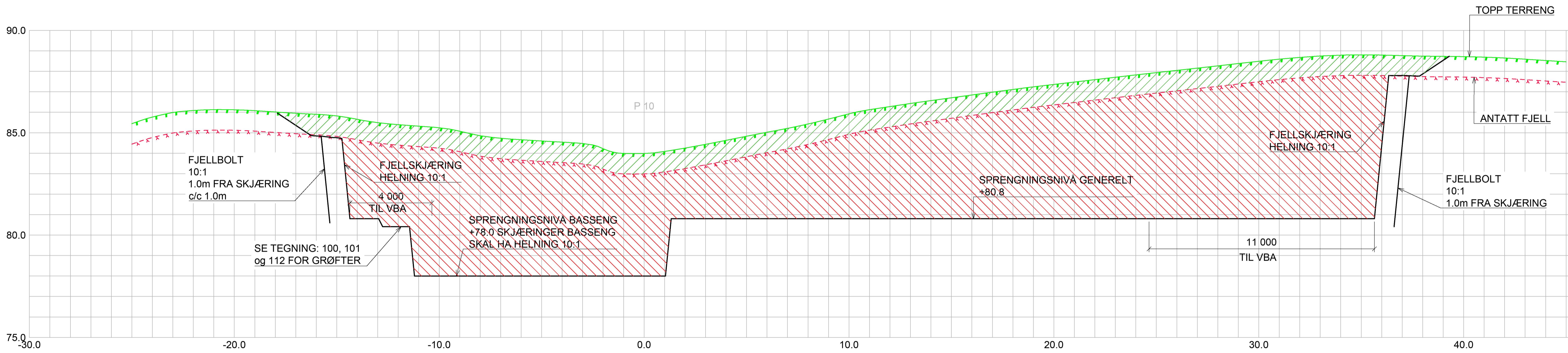
SNITT A-A - FRA TEGN 200 M = 1:100
