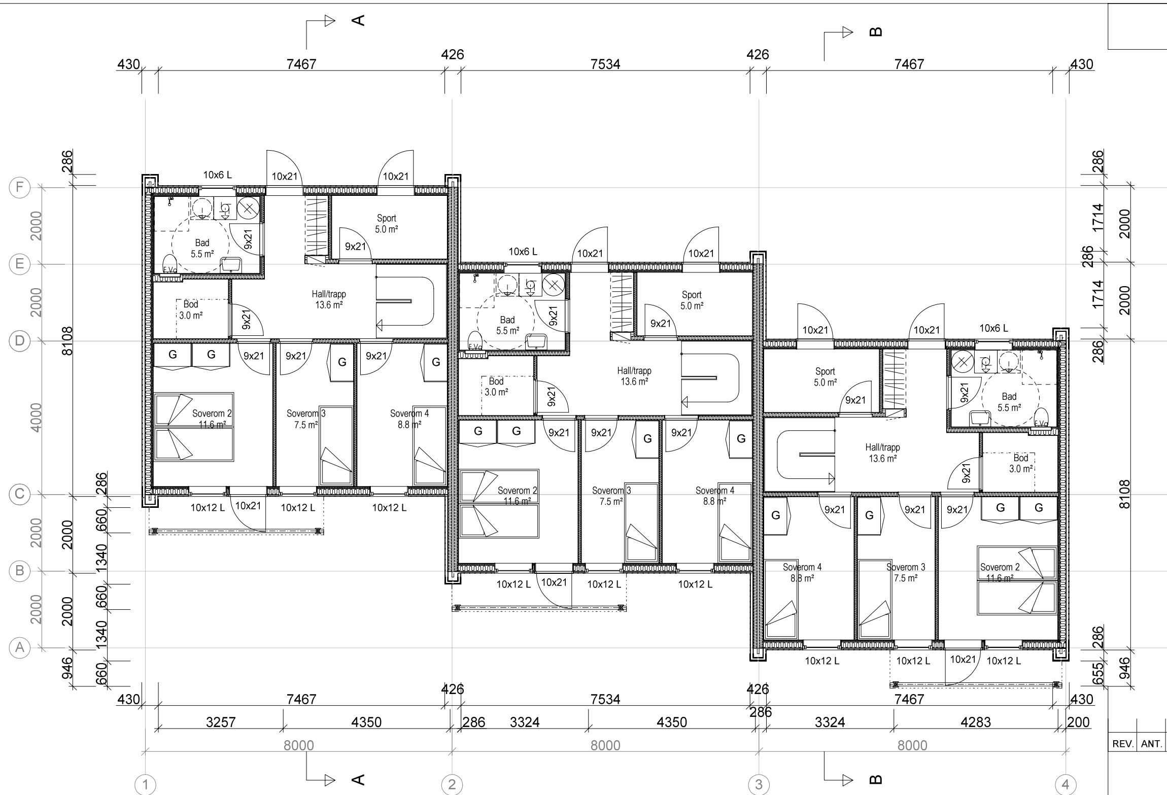
BOLIG 38: Plan 1. etasje BRA 58,1 m2
