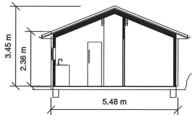
SNITT A-A
