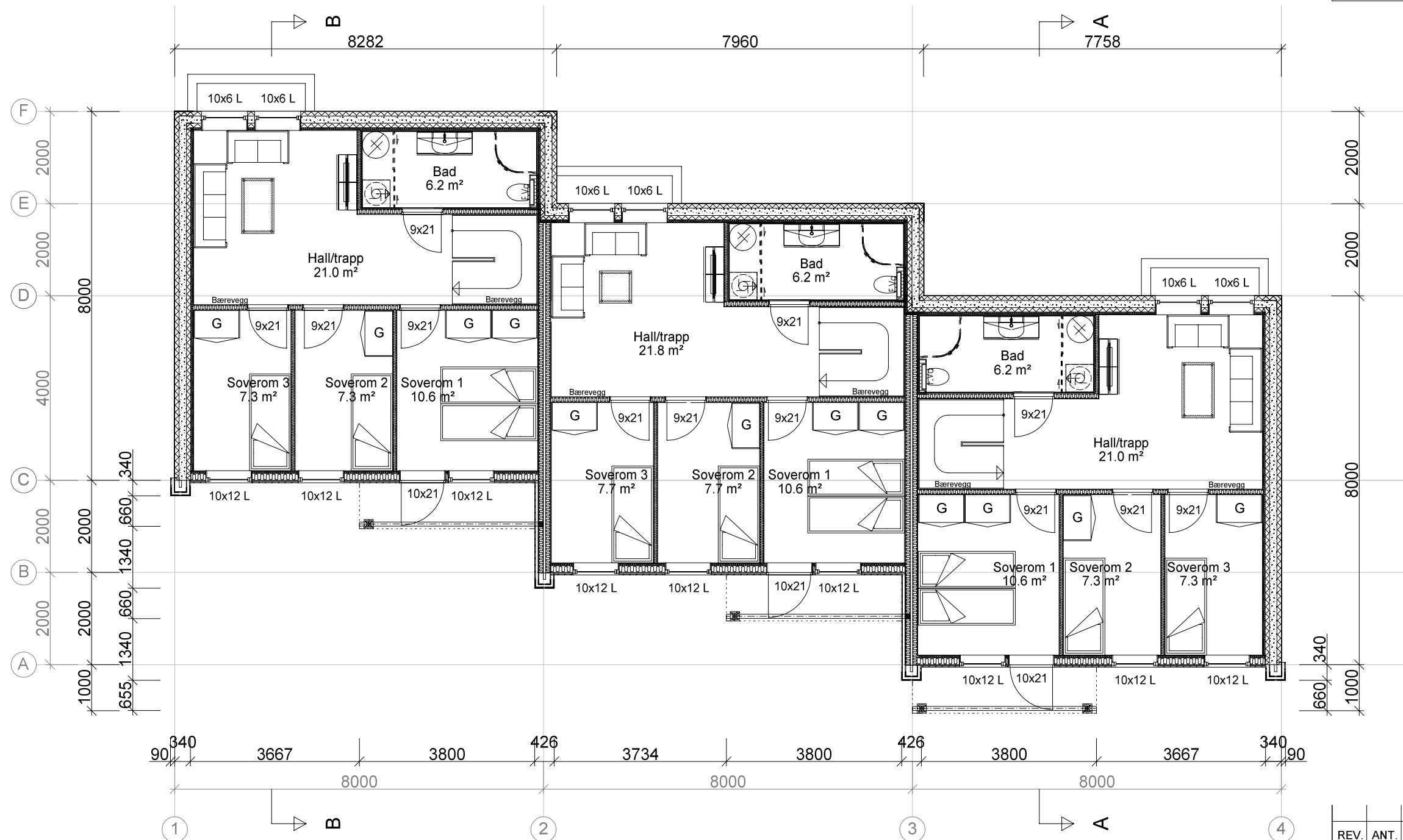
BOLIG 44 Plan U. etasje BRA 55,1 m 2
