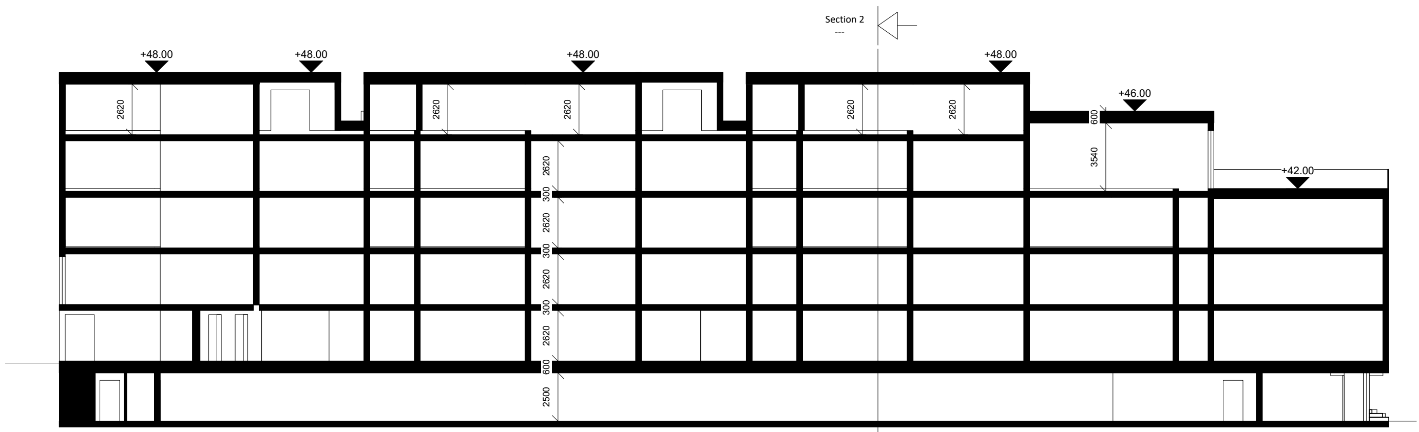
Prinsippsnitt Bygningskropp mot nord
