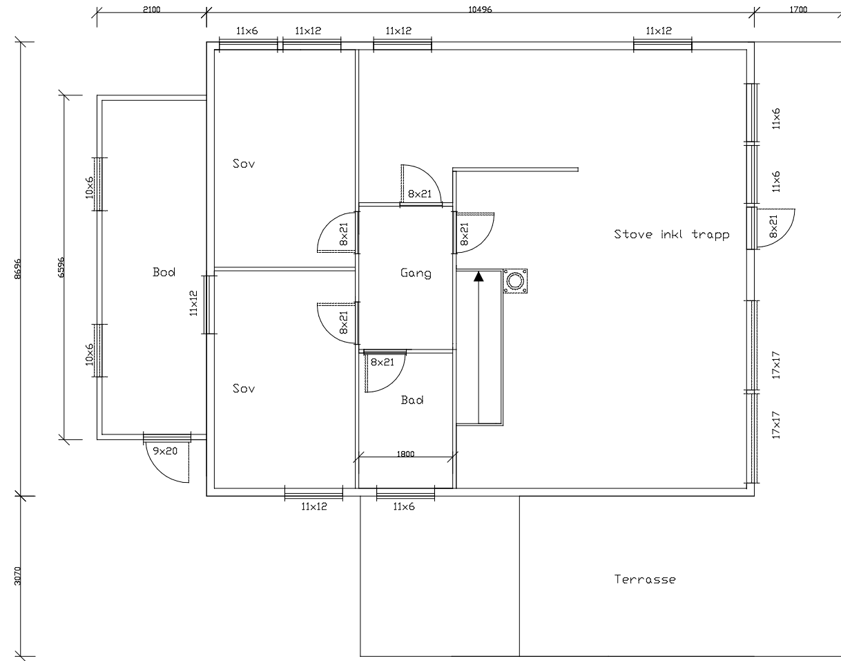
Plan hovedetasje
