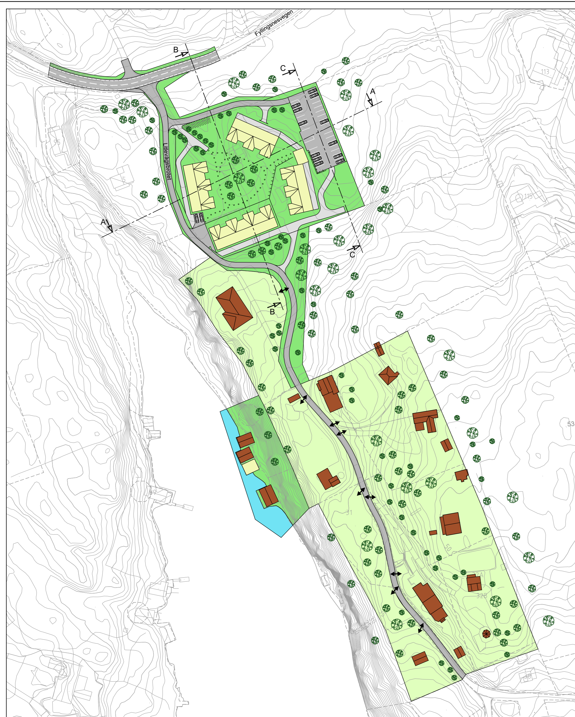
Utsnitt M=1:500
