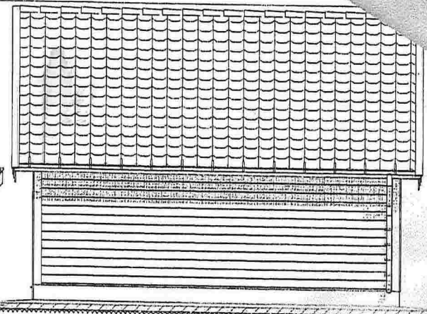
Fasade 3 1:100
