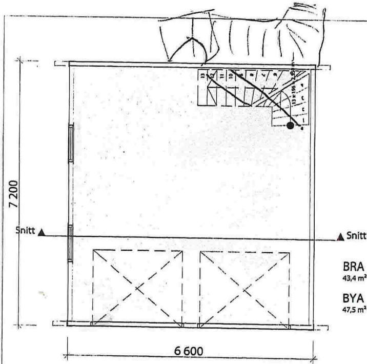
Plan 1 etasje 1:100
