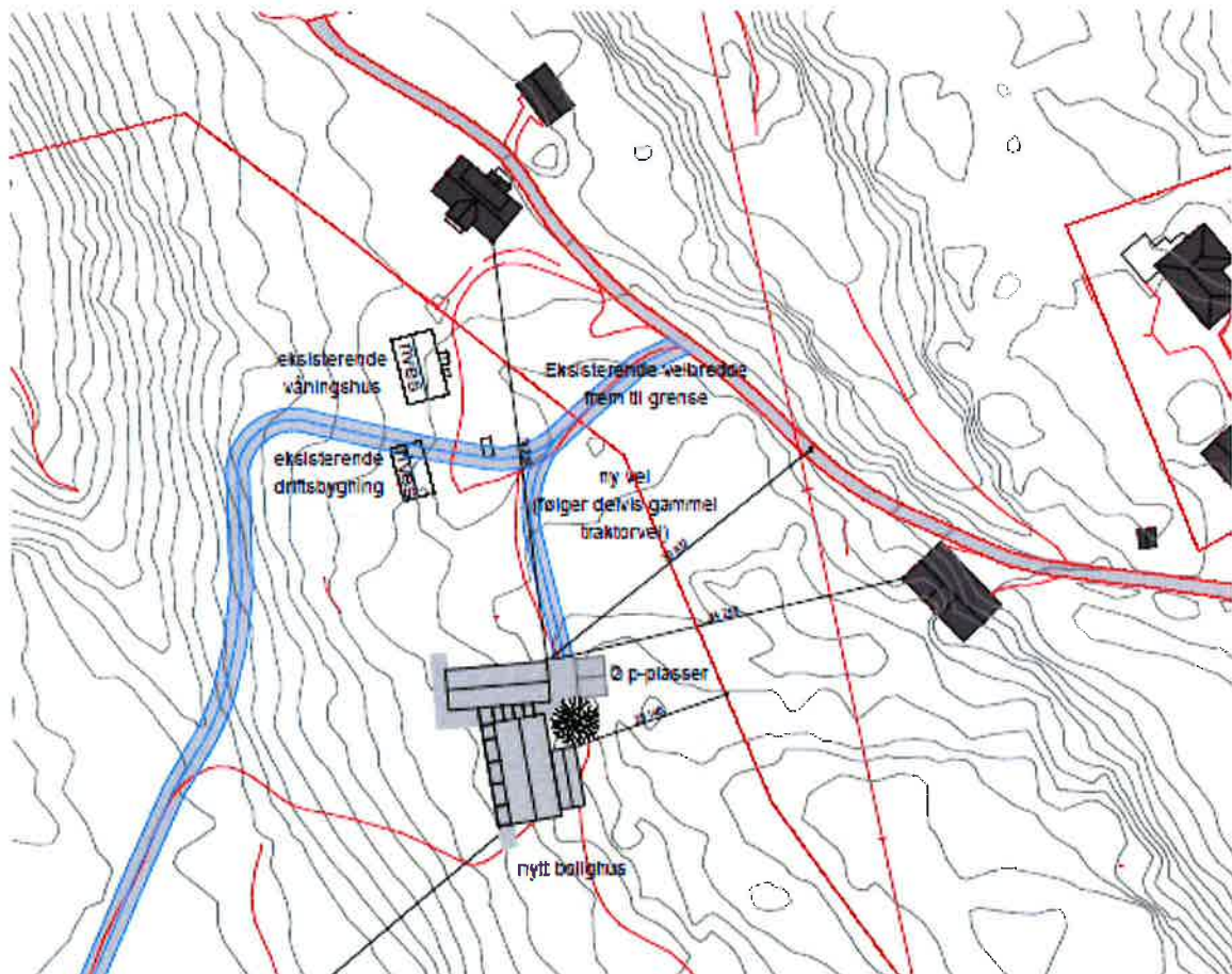
Planskisse fra søknaden. Vegtraséen er justert noe iht. plantegning i vedlegg 1.
