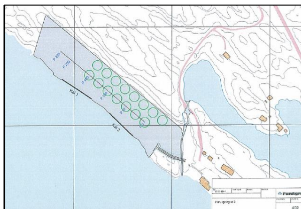
Figur 3. Det foreligger to nokså like alternativer for utvidelse av settefiskanlegget. I alternativ 2 (t.h.) beholdes vannstrengen fra Kjøggjarvatnet til sjøen åpen, mens den i alternativ 1 (t.v.) legges i rør/kulvert (kilde: FanAgro AS).
