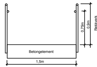
Tverrprofil
