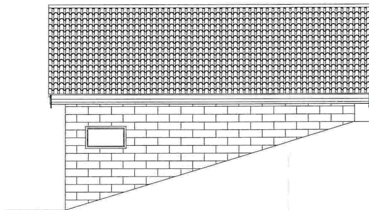
Fasade mot:Øst
