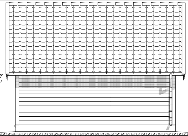
Fasade 3 1:100
