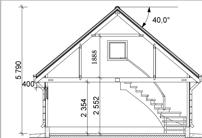
Snitt 1:100
