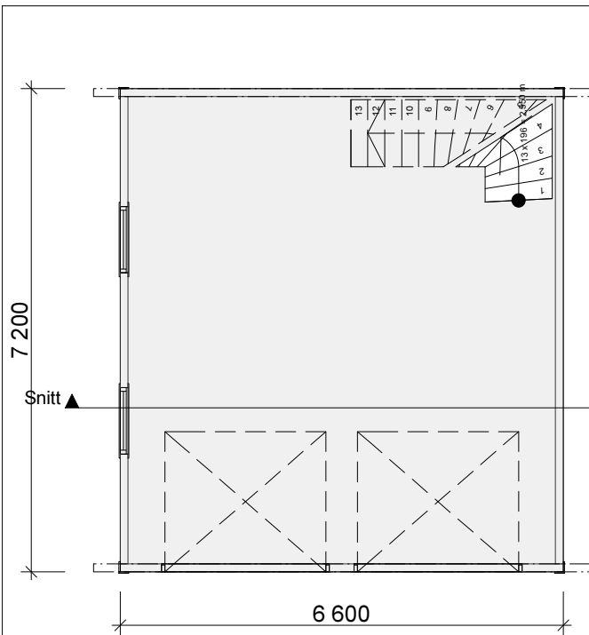
Plan 1 etasje 1:100
