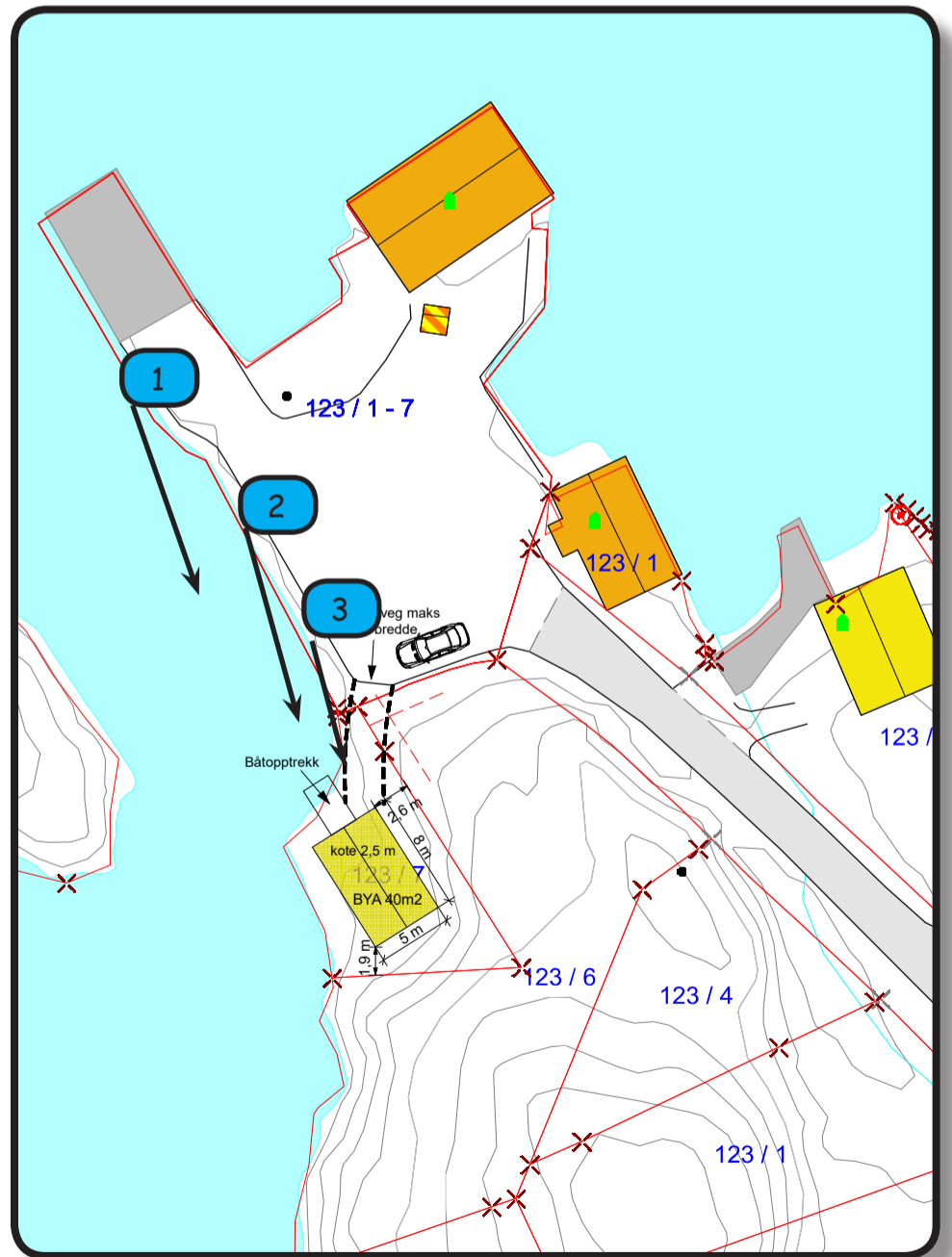
Situasjonsplan
