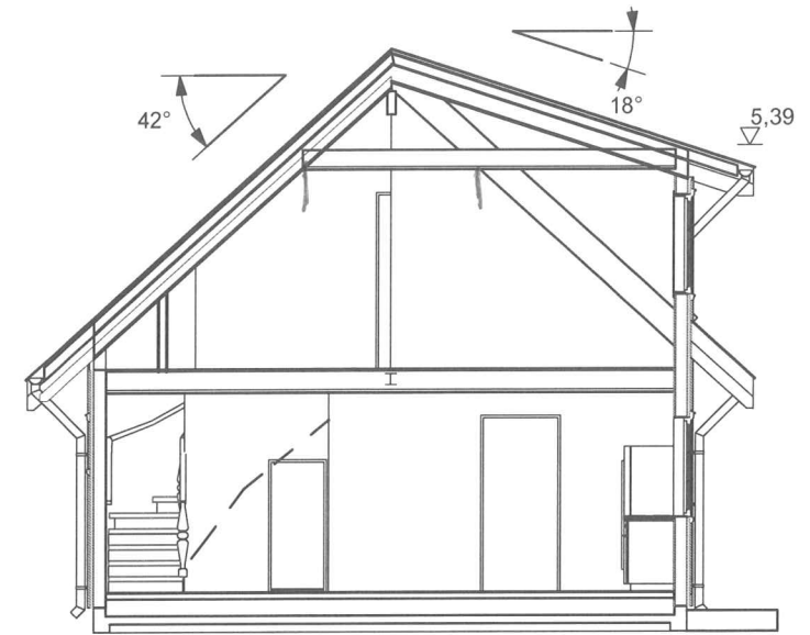
SNITT A-A
