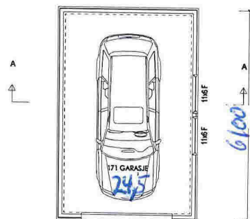
HOVEDPLAN
