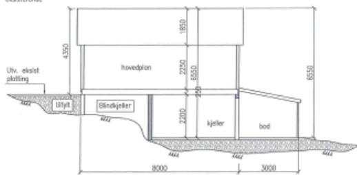
Snitt A-A eksisterende
