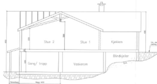
Snitt C-C Etter endring
