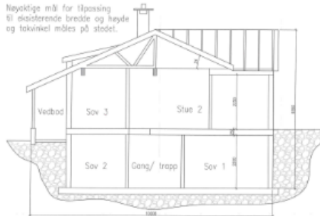
Snitt C-C Etter endring
