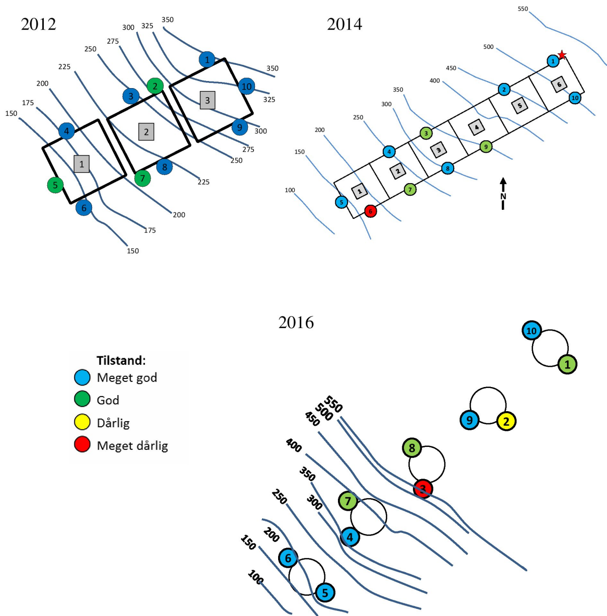
Figur 6. Oversikt over MOM B-tilstand (middelverdien av gruppe II og III parametrar) for dei 10 grabbhogga som vart tekne på lokaliteten Langøy ved granskinga 25. mai 2012 (Furset 2012) (oppe), 6. juli 2014 (Tverberg mfl. 2014) (midten) og noverande gransking 27. januar 2016.
