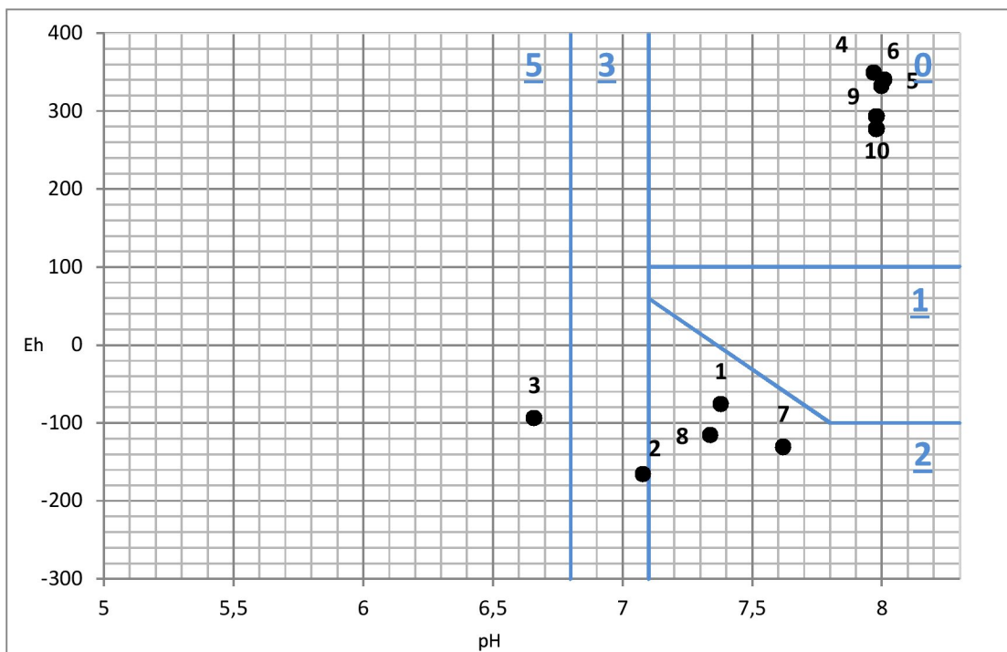
Figur 5. Forholdet mellom elektrodepotensial (Eh) og surleik (pH) for 10 grabbhogg (nummererte punkt) tekne 27. januar 2016 ved Langøy. Poengkategoriar med støttelinjer for gruppe II-parameteren er markert (NS 9410:2007).
