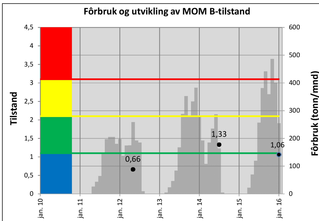
Figur 7. Fôrforbruk (grå stolpar) og utvikling av MOM B-tilstand (svarte punkt) ved lokaliteten Langøy i Lindås kommune sidan 2011. Anlegget i 2011 besto av tre bur, og vart utvida med ytterlegare tre bur før utsettet våren 2013, og i 2015 vart anlegget endra til fem 160 m ringar med lengre utstrekning.
