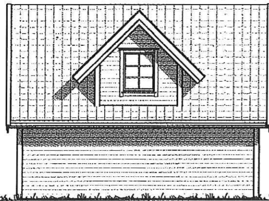
FASADE 1
