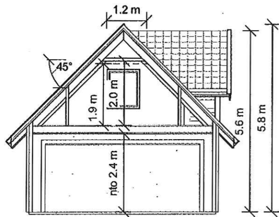
SNITT A-A
