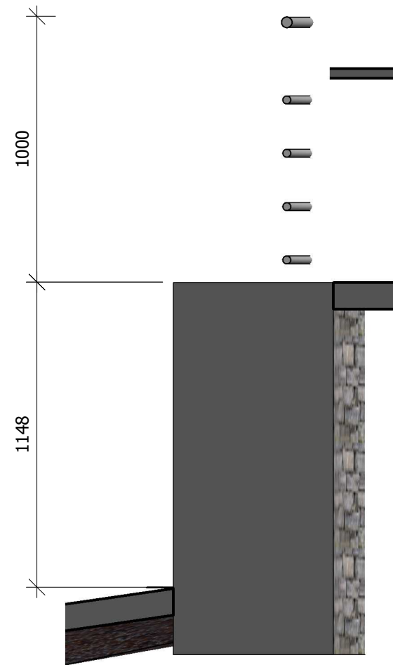
Snitt C-C 1 : 20
