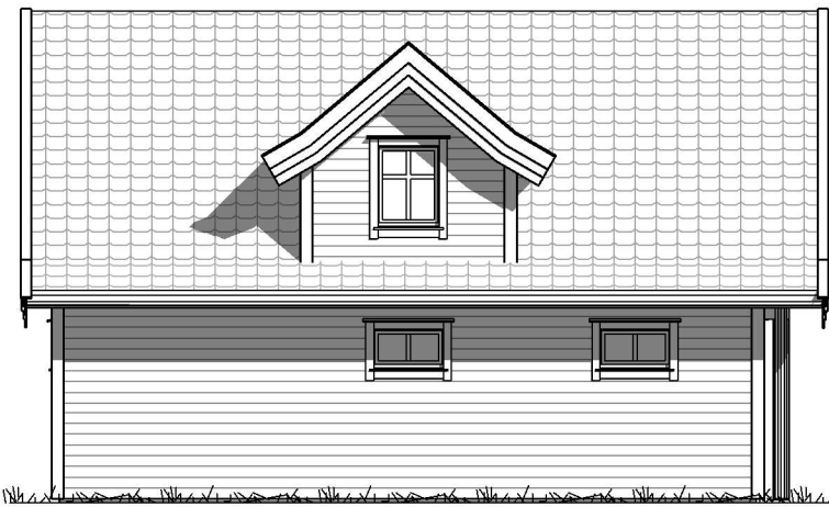
FASADE 1
