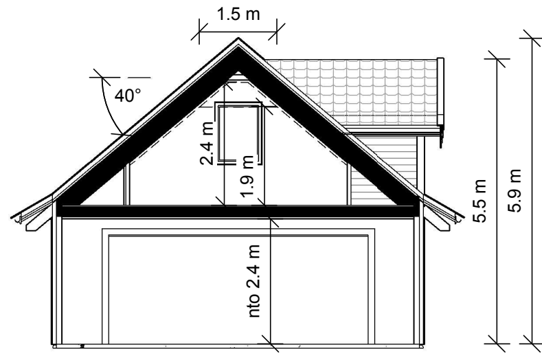
SNITT A-A
