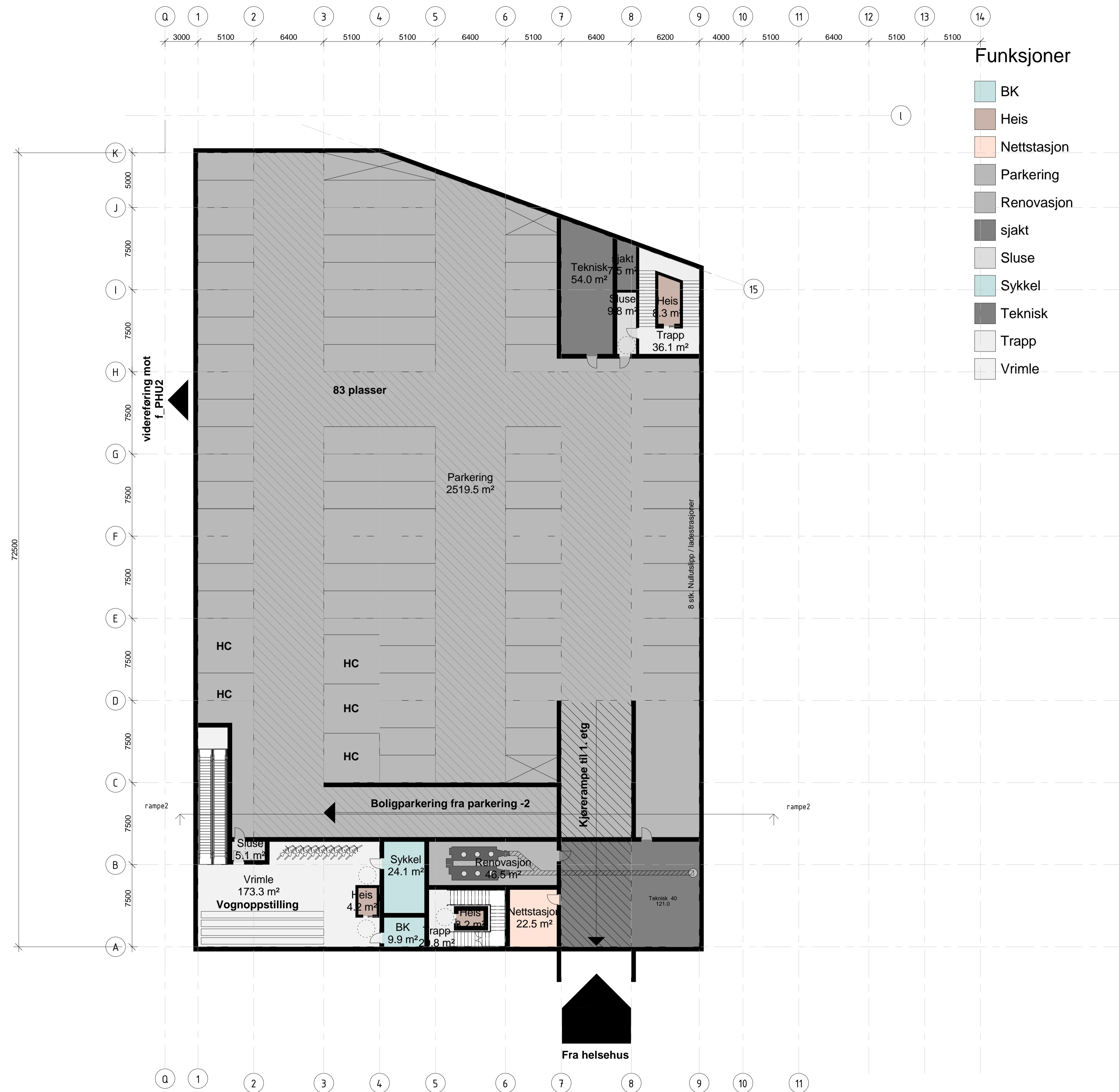
-1. parkdekke 1 : 200
