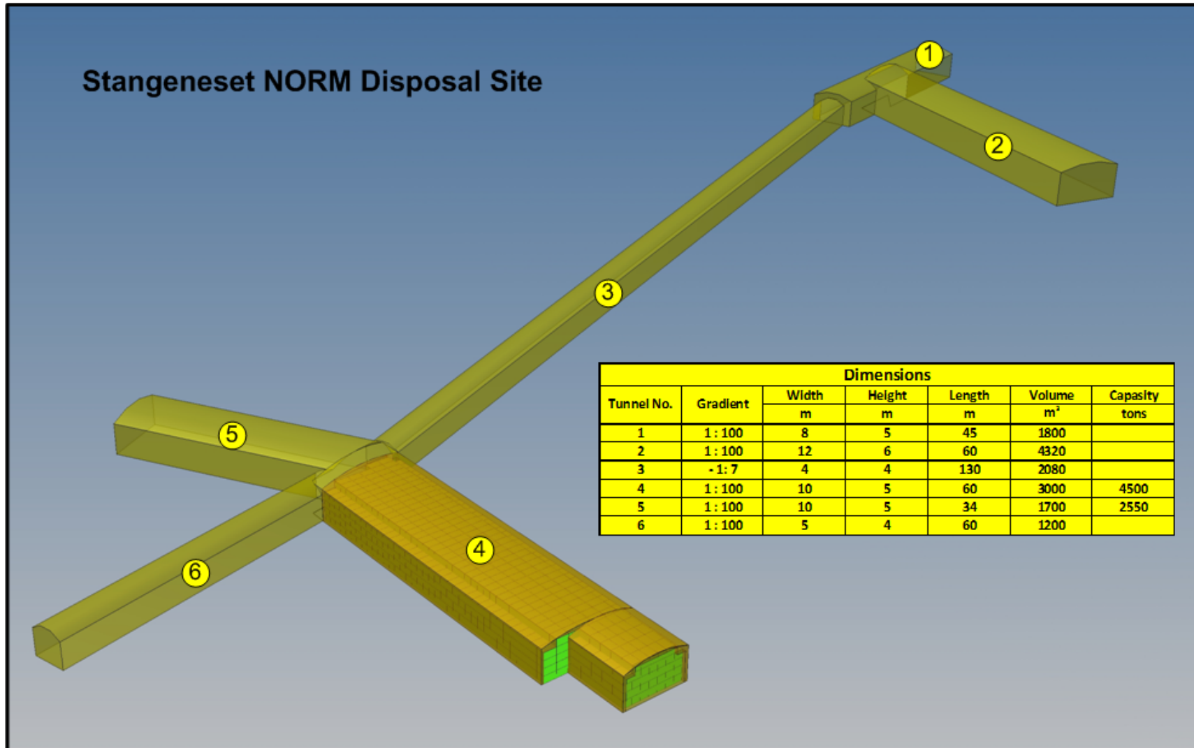
Vedlegg 1: Skisse av deponianlegget med angivelse av tunneller, volum og kapasitet.
