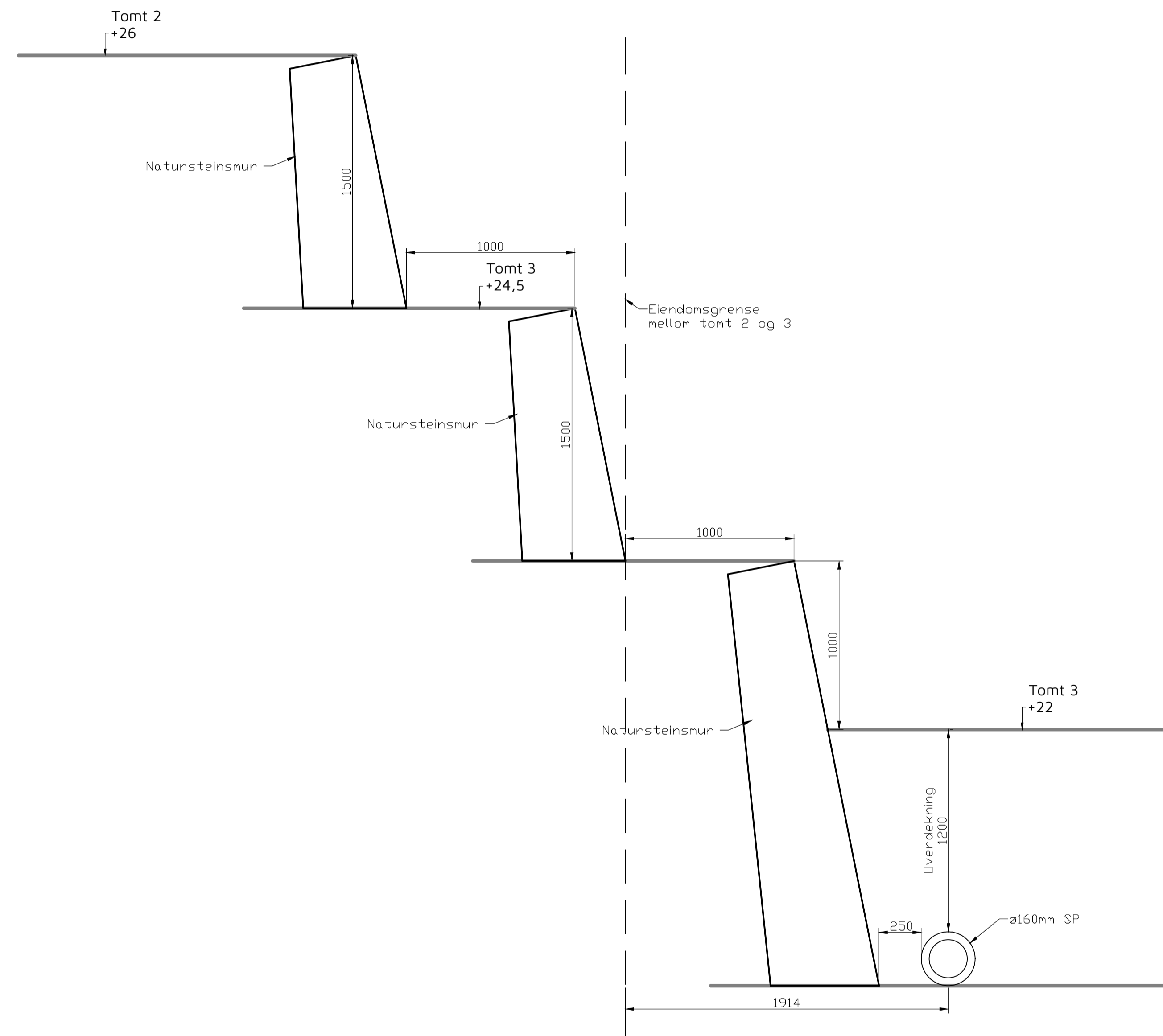
SNITT MUR MELLOM TOMT 2 OG 3. M=1:20
