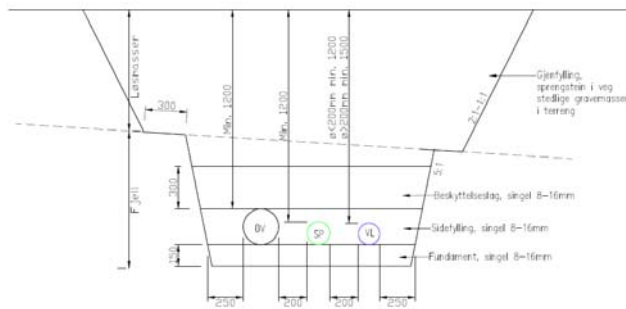
TYPISK GRØFTESNITT. M=1:20 Vann-, spillvann- og overvannsledning
