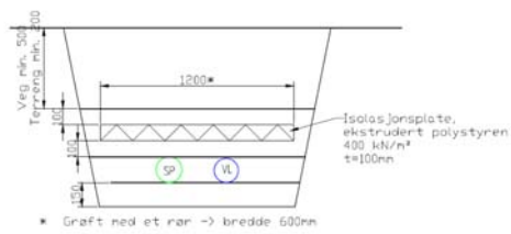
GRØFTESNITT. M=1:20 Grunn, isolert grøft
