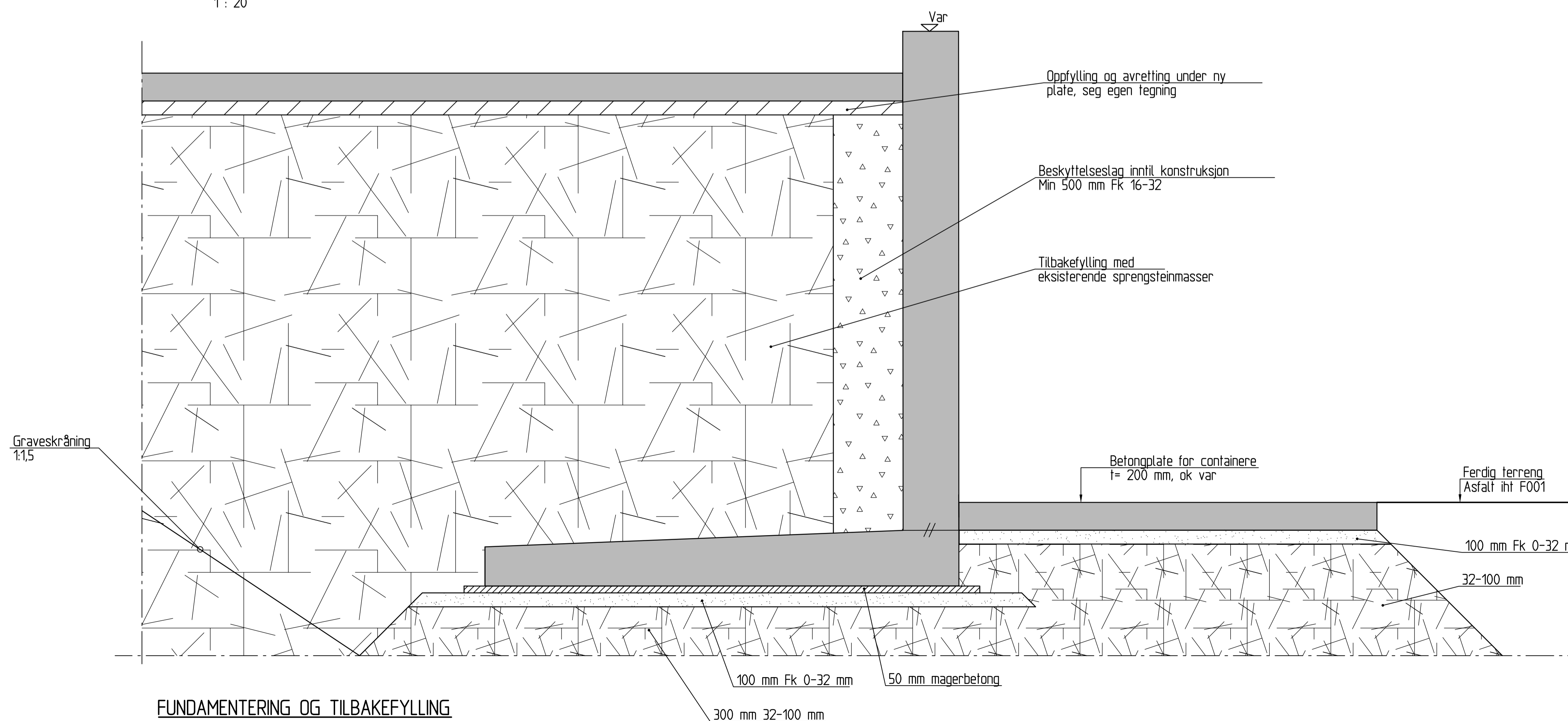
SNITT A-A K152 1 : 20
