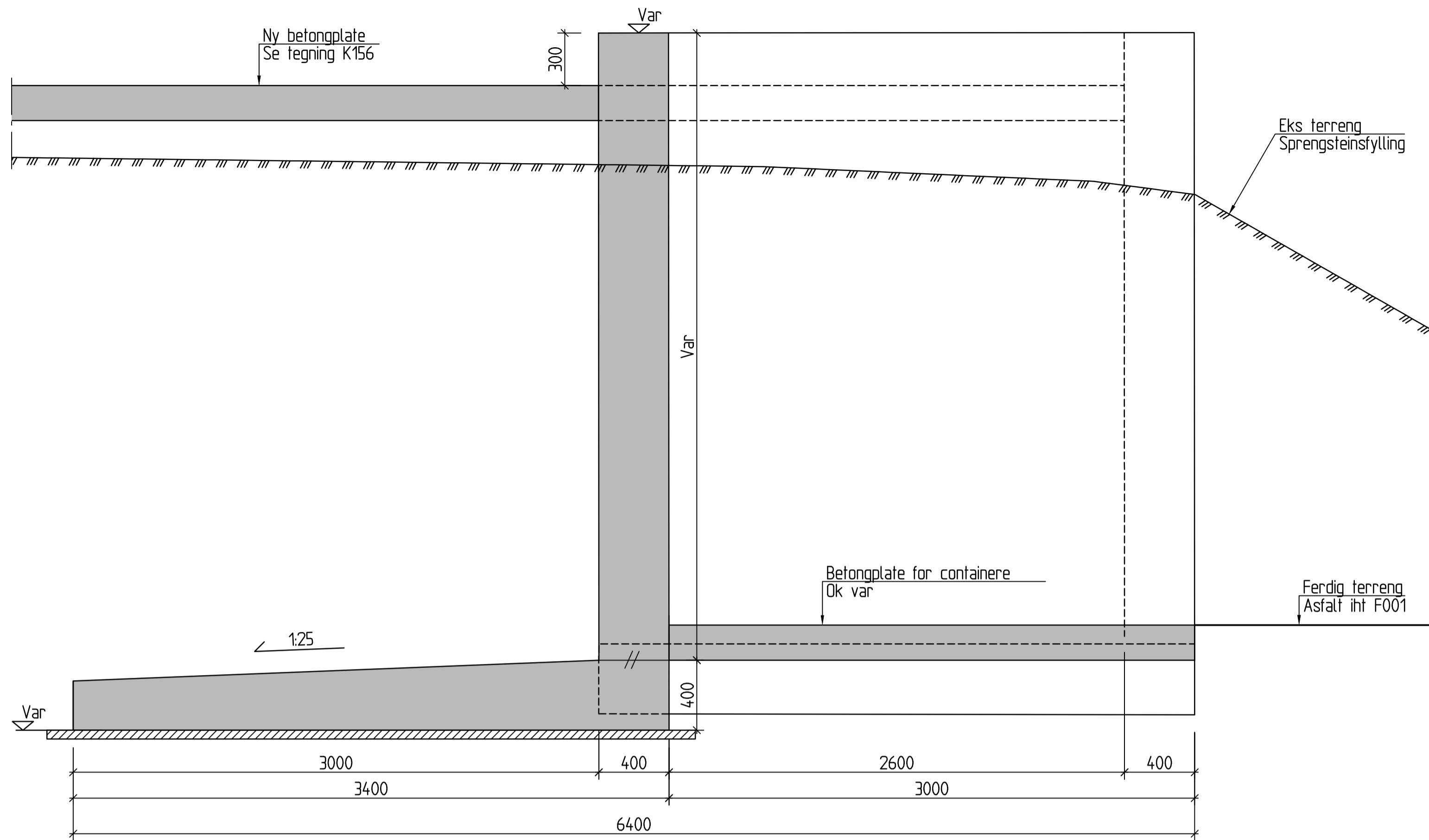
SNITT B-B K152 1 : 20
