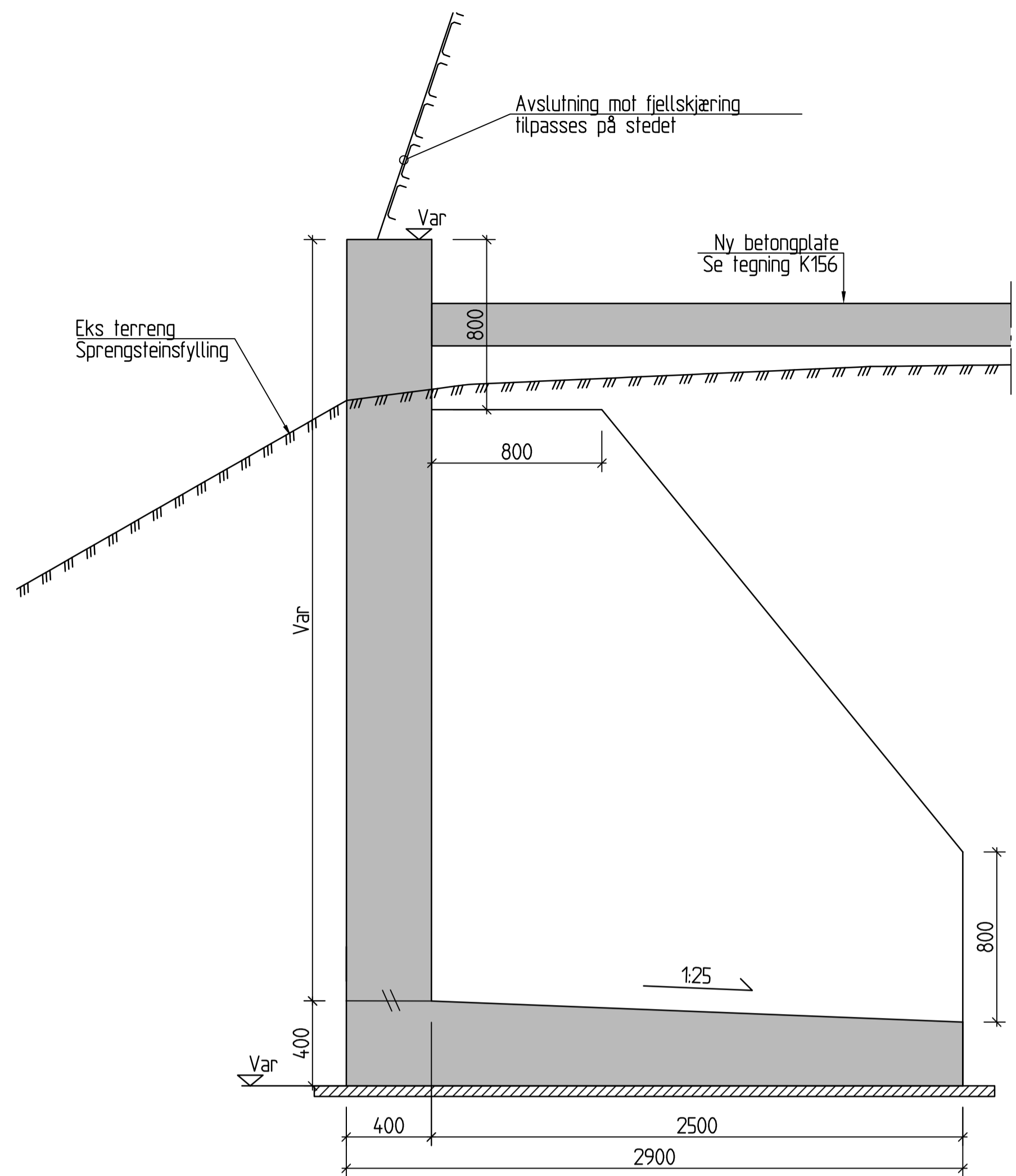
SNITT A-A K152 1 : 20
