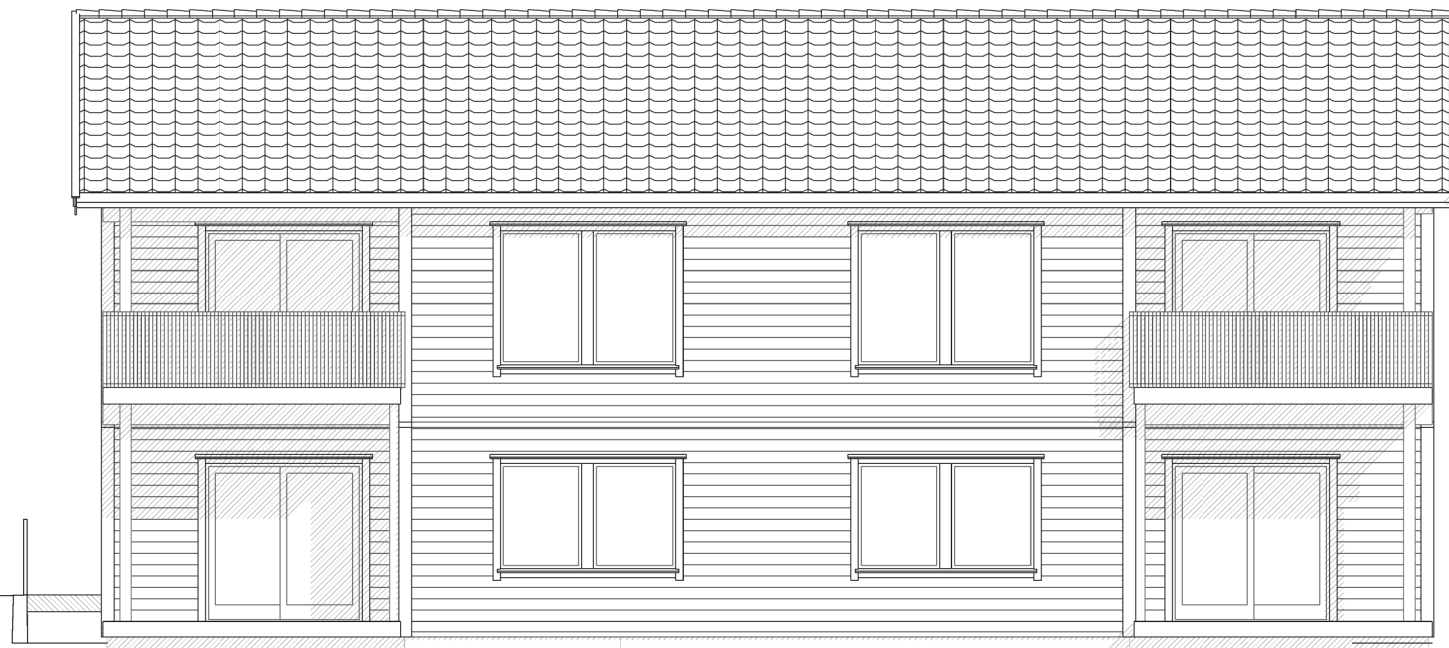
FASADE SØR
