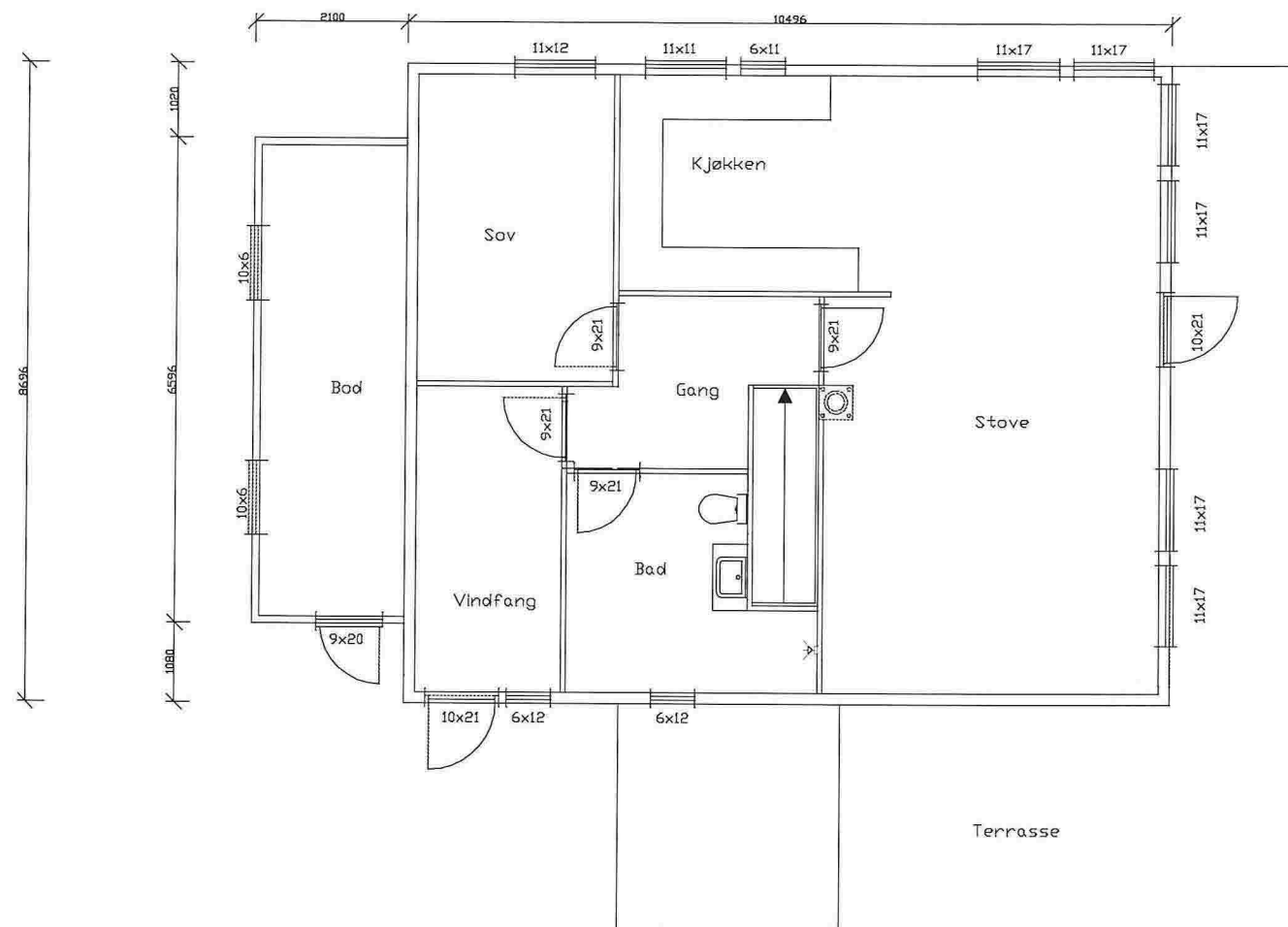
Plan hovedetasje
