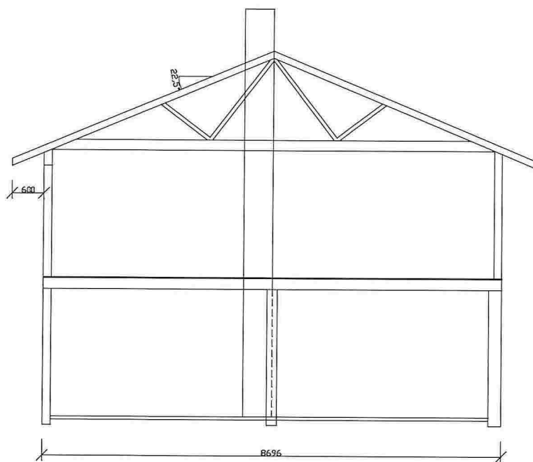
Snitt
