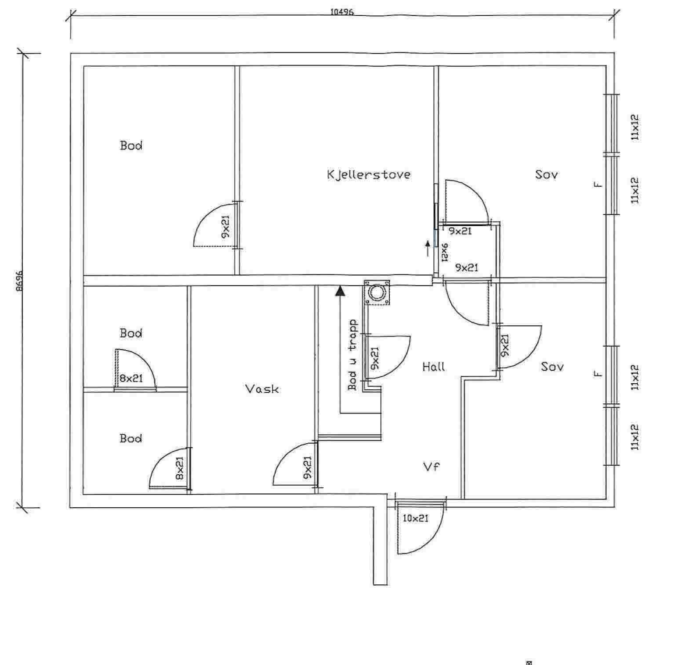
Plan underetasje
