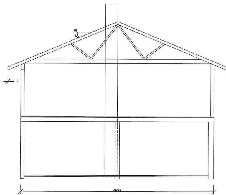
Snitt
