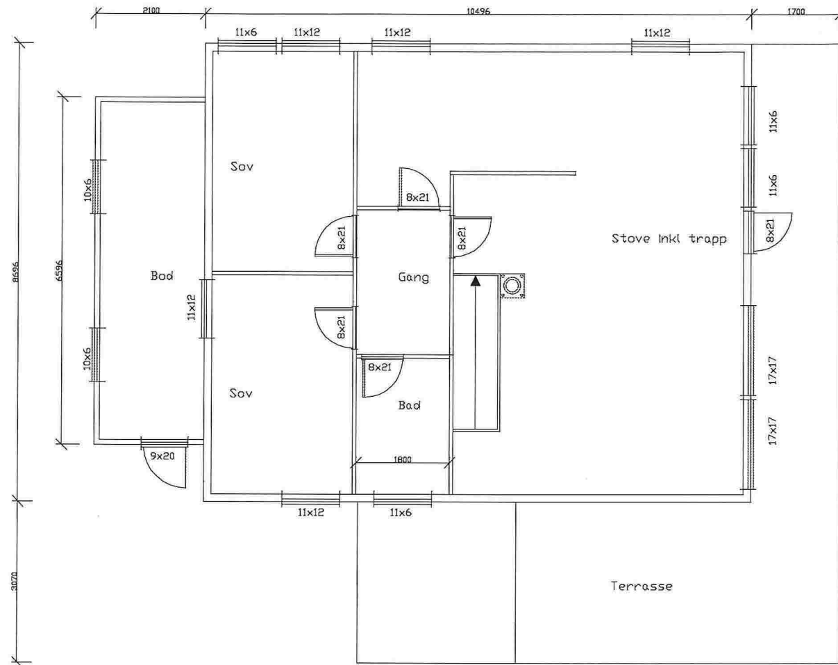
Plan hovedetasje
