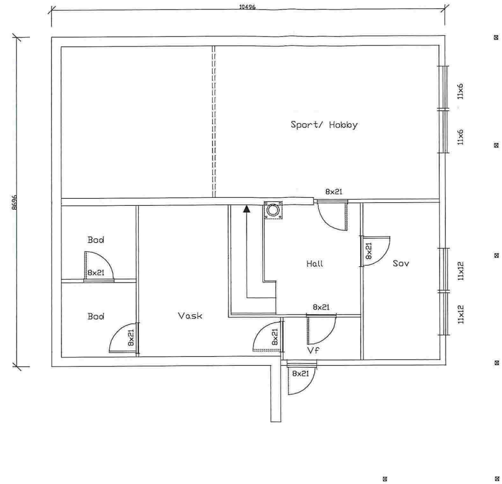
Plan underetasje
