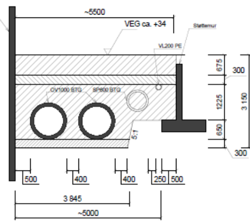
Grøftesnitt 3 - Ved nedkøyringsrampe helsehuset
