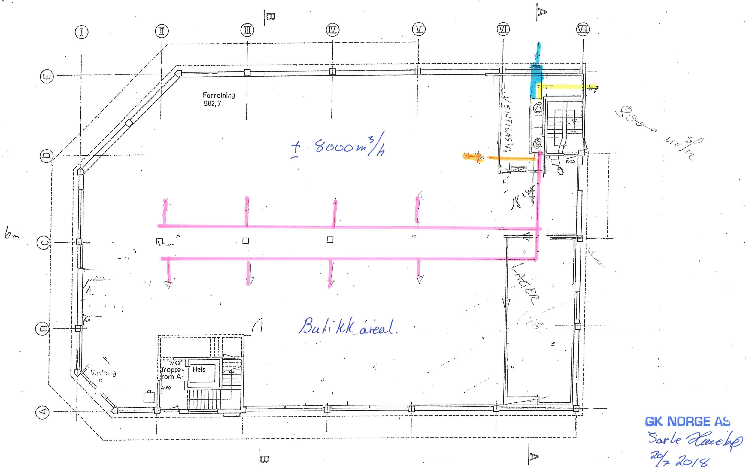
PLAN 1. ETG.
