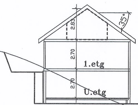
Snitt hustype1 med u.etg. + 1.etg. Tomt nr. 48, 58, 59, 60, 64, 65, 66, 67, 68, 69, 75, 76, 77, 79, 92
