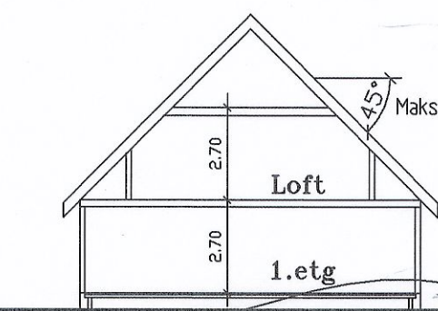
Snitt hustype2 med 1 etg + loft Tomt nr. 49, 54, 55, 56, 62, 63, 70, 71, 81, 82, 83, 91
