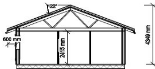
Snitt 2 1 : 100
