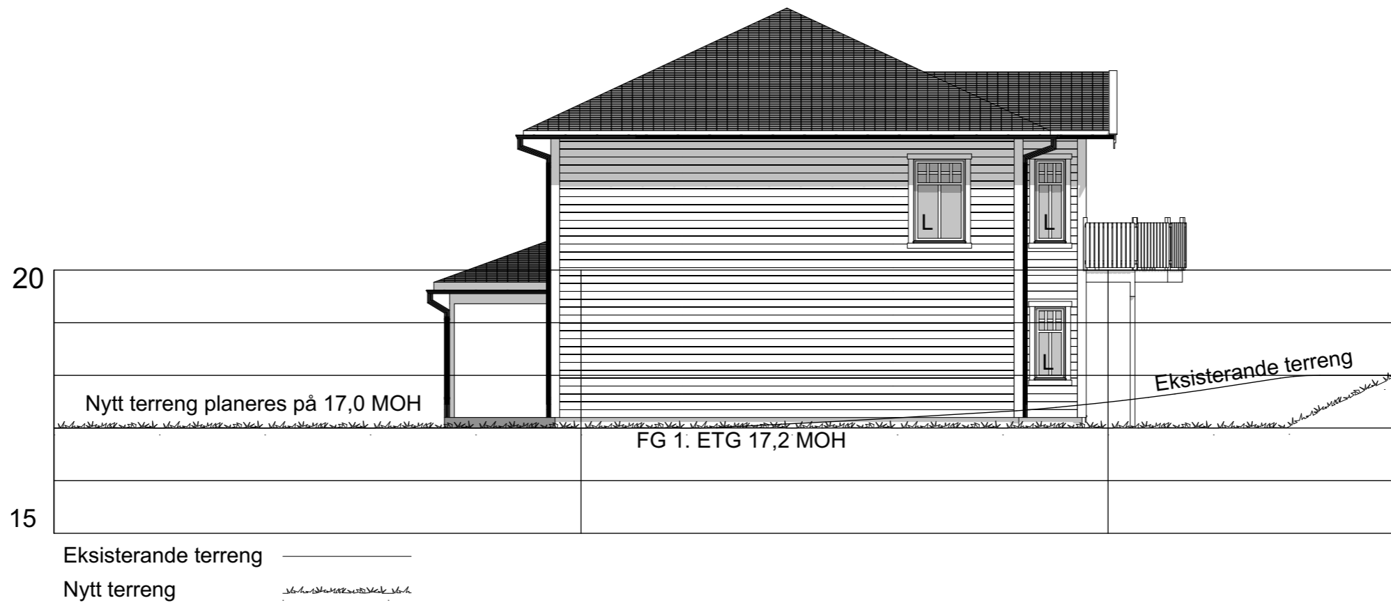
Fasade 4 Nord-Øst
