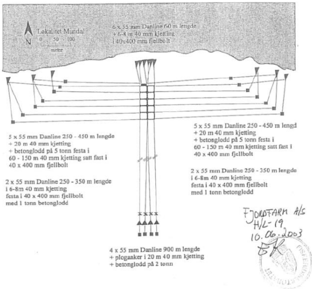
Figur 4.3. Plassering av anlegget med fortøyningsplan ca 90 m frå land ved Mundal teikna etter økonomisk kartverk ( M=1:5\ 000 ). Kartreferanse, sjokart: N 60°33,82' E 05°21,54'.
