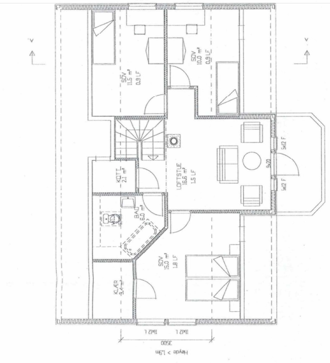
LOFTPLAN
