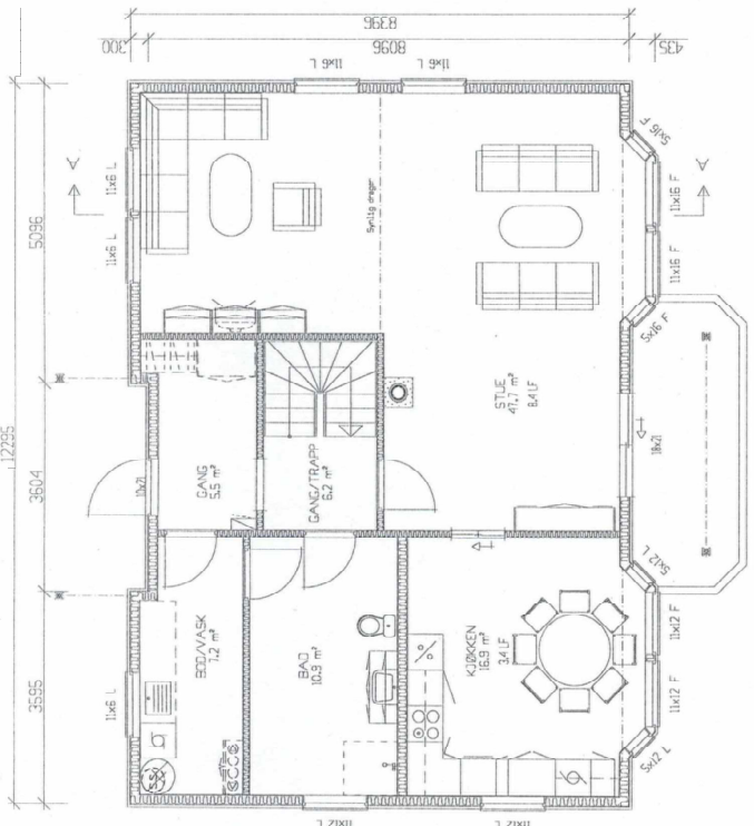
HOVEDPLAN
