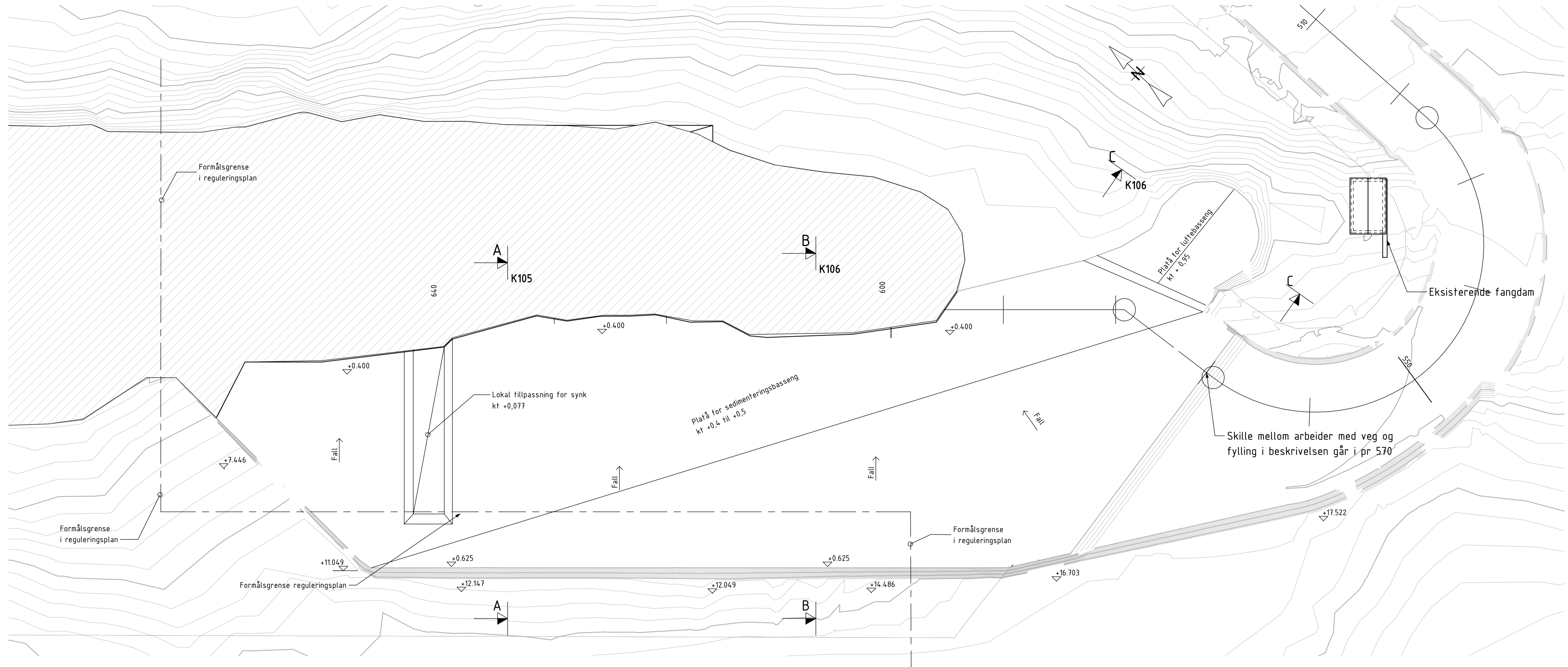
Sprengingsplan 1 : 200
