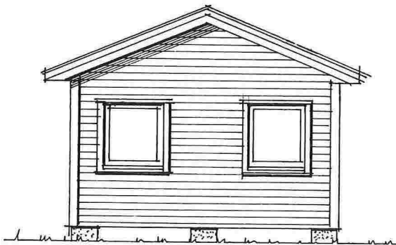
Fasade mot NØ
