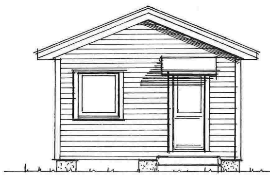
Fasade mot SV
