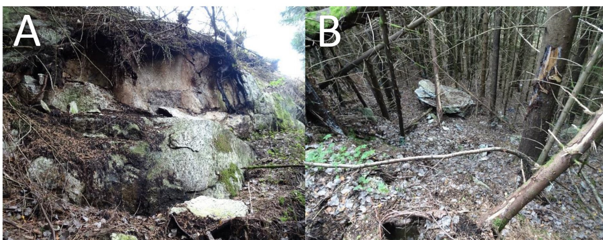
Figur 4. A) Løsneområde for relativt ferskt steinsprang. Merk de mørke røttene som vokser på utsiden av det ferske bruddet. Bildet er tatt mot øst. B) Steinsprangblokk på om lag 2 m 3 . Bildet er tatt mot sørvest.
