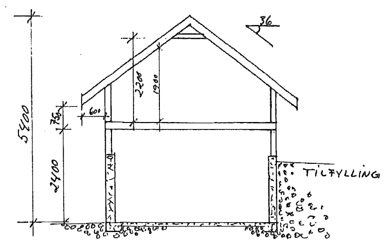
SNITT A-A
