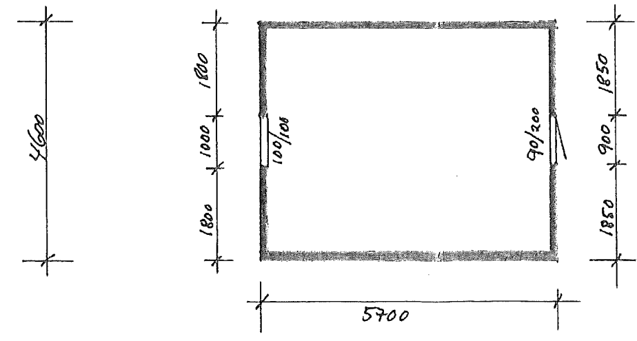
LOFT PLAN
