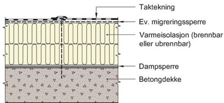
Figur 31 - Rettvendt tak med bærekonstruksjon av betong (SINTEF Byggforsk)
