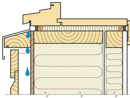
Figur 21 - Vindu plassert med sporet i bunnkarmen for sålbenbeslaget i plan med vindspærren (SINTEF Byggforsk)
