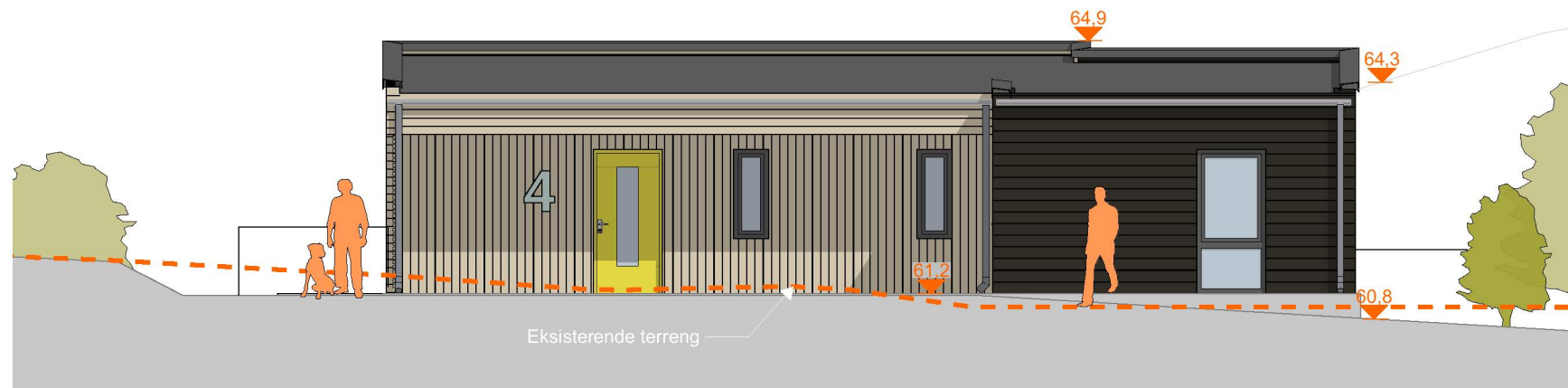
1:100 Fasade Nord
