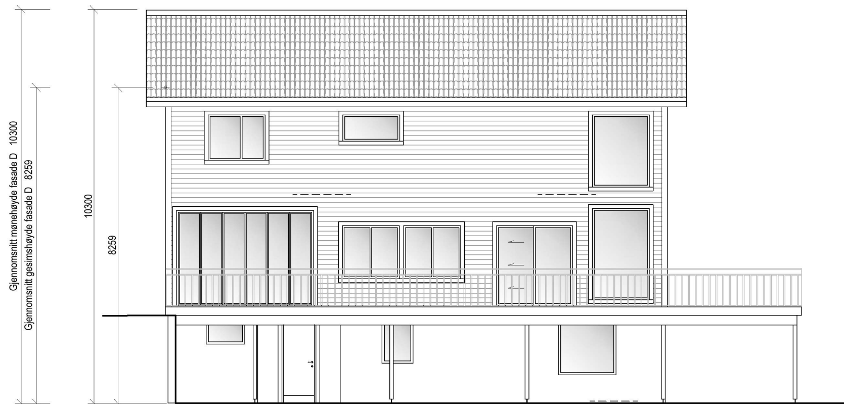
D, FASADE MOT SØRVEST
