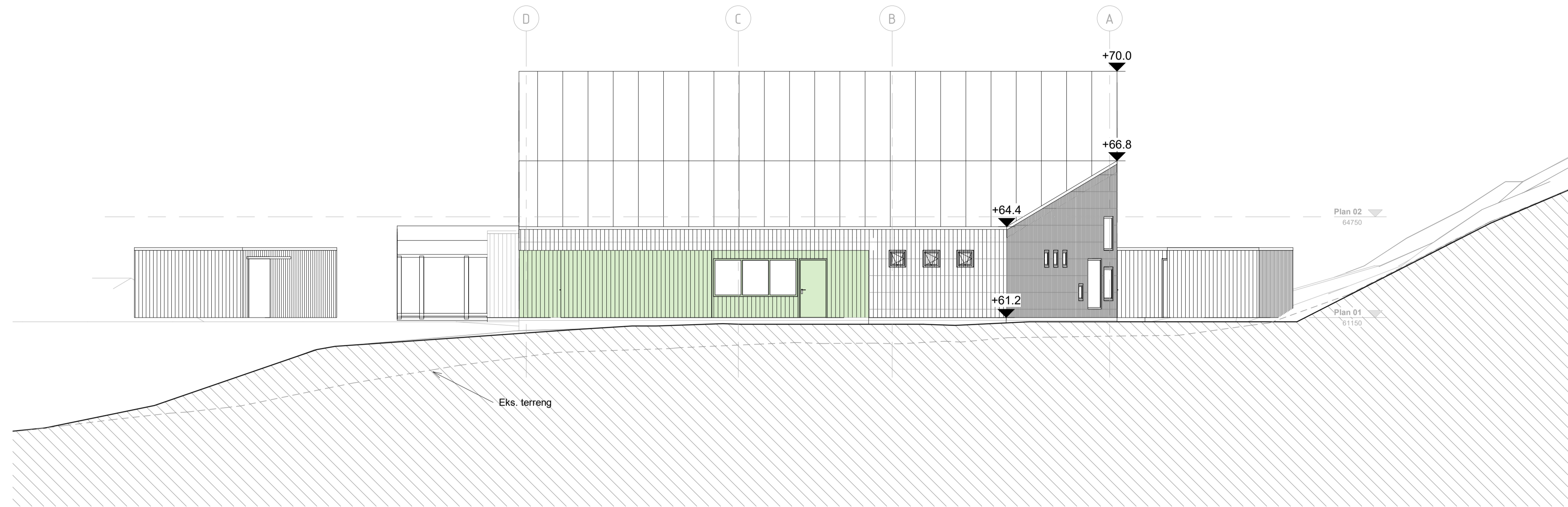
Fasade mot nord 1 : 100
