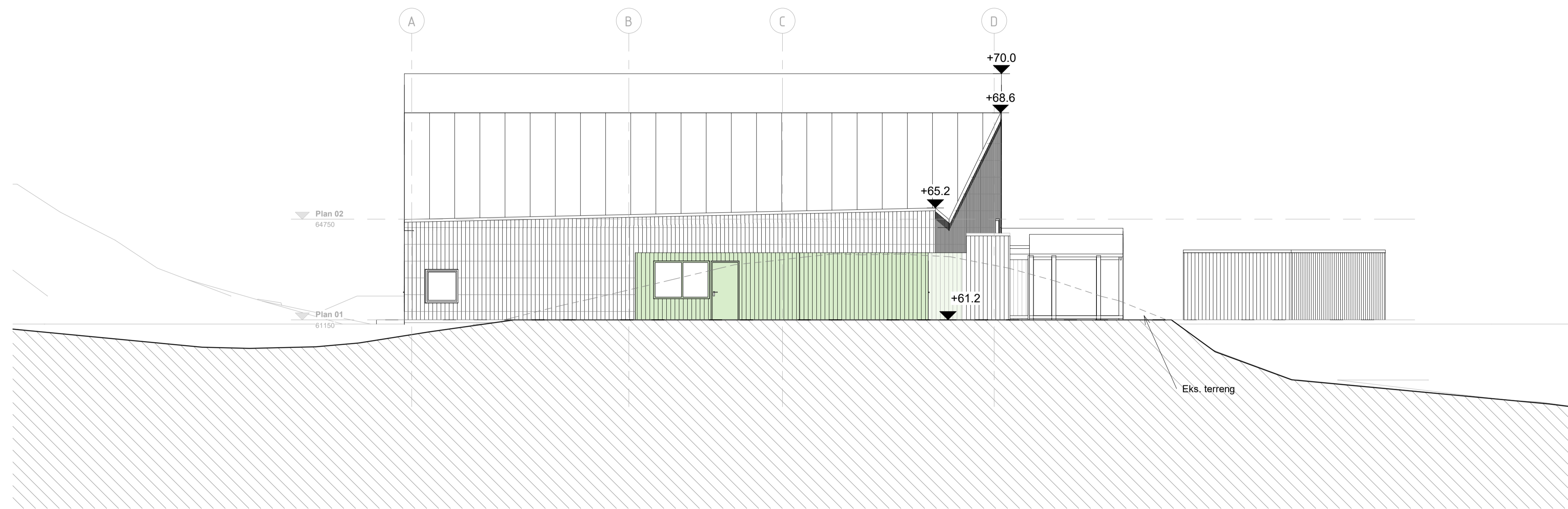
Fasade mot sørvest 1 : 100
