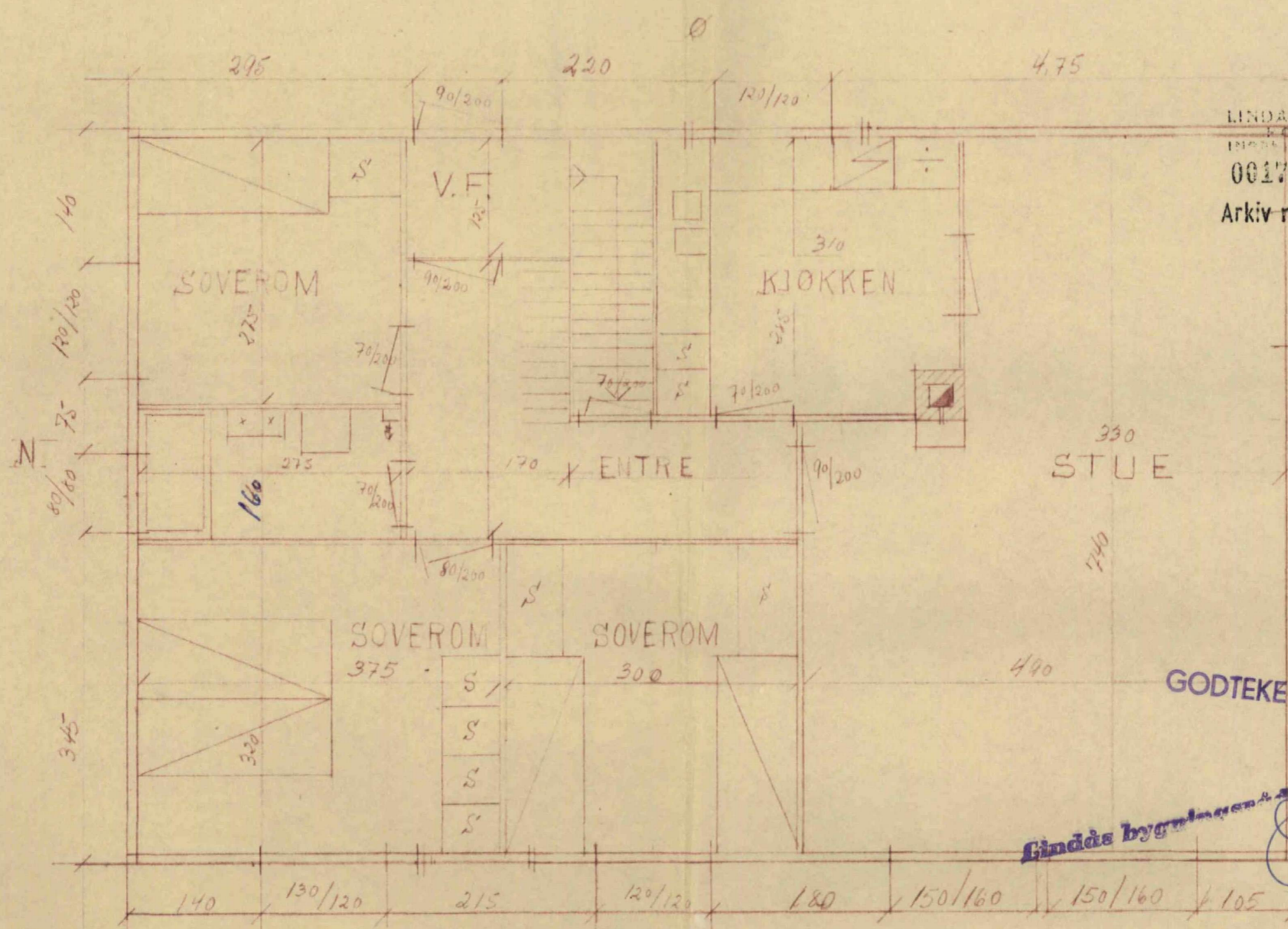
ETASJEPLAN MAAL 1-50
