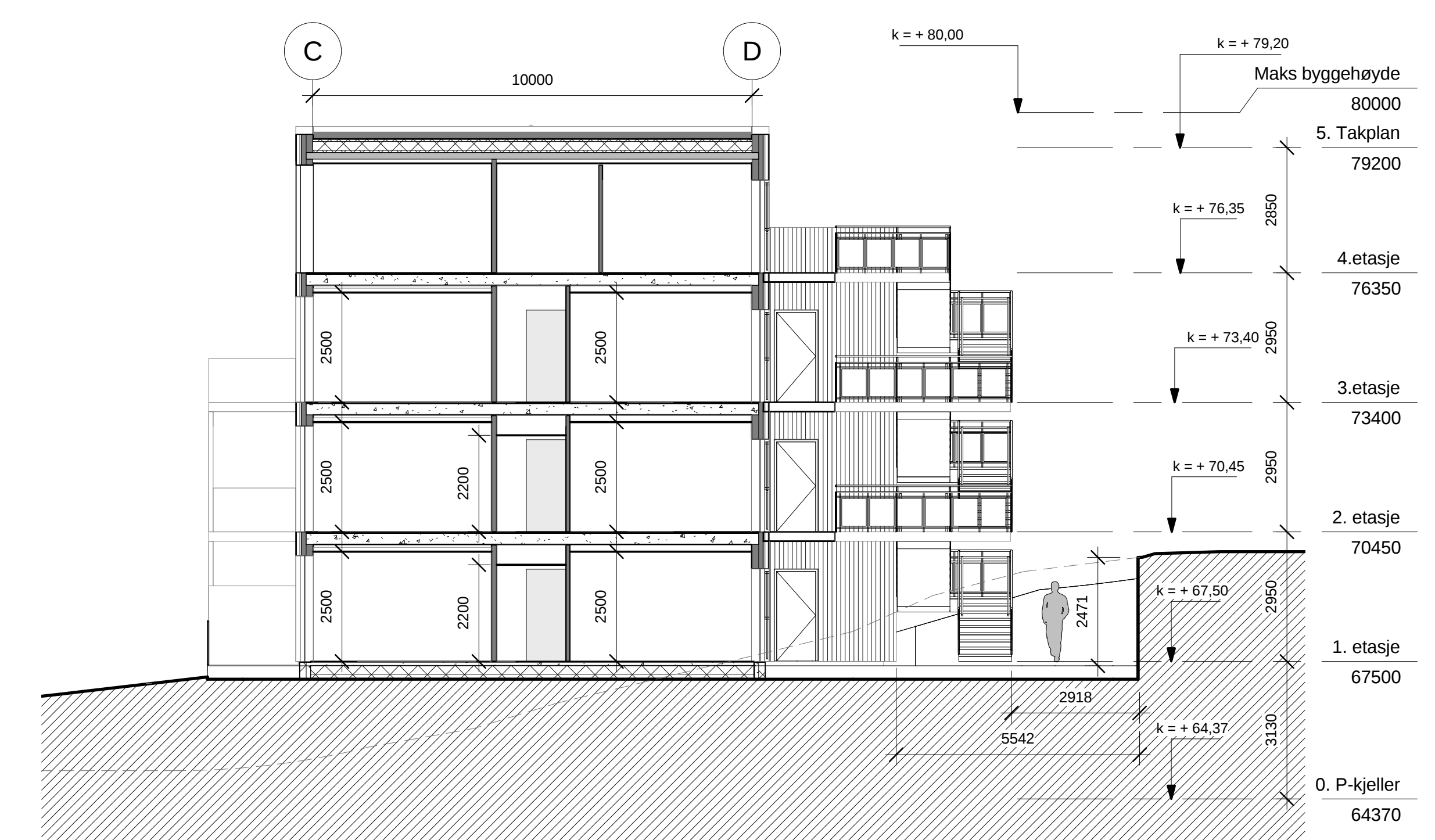
3 Snitt Hus C 1 : 100
