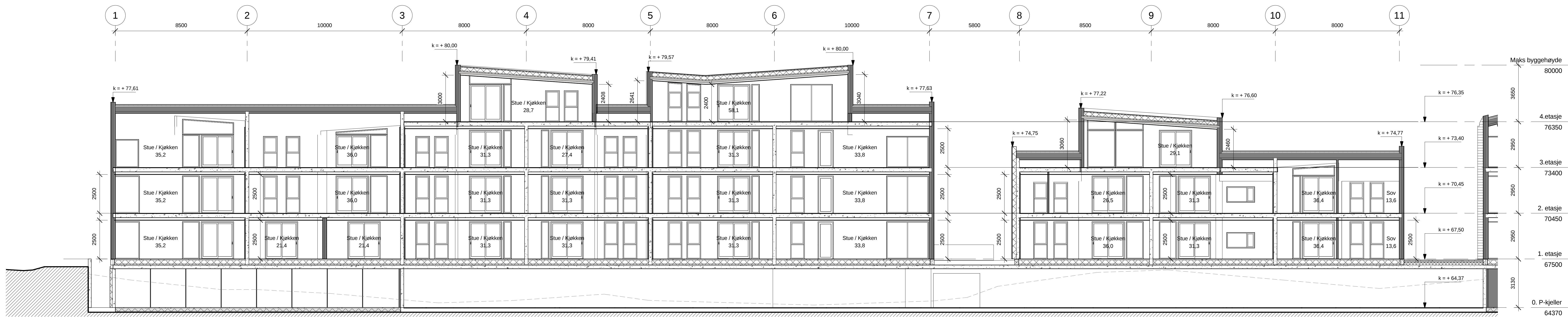
1 Langsnitt Hus A og B 1 : 100
