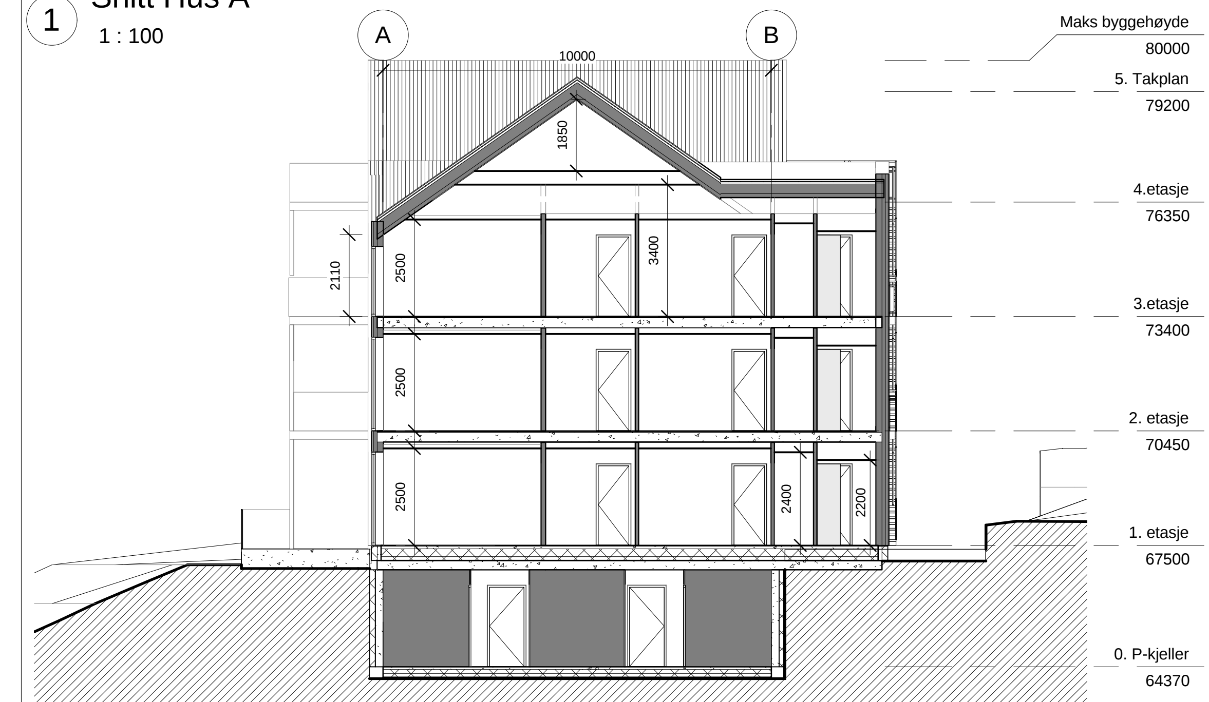
4 Snitt-A04 1 : 100
