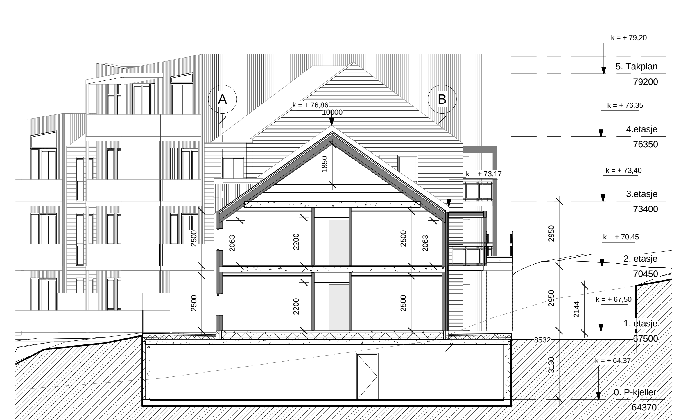
2 Snitt Hus B 1 : 100
