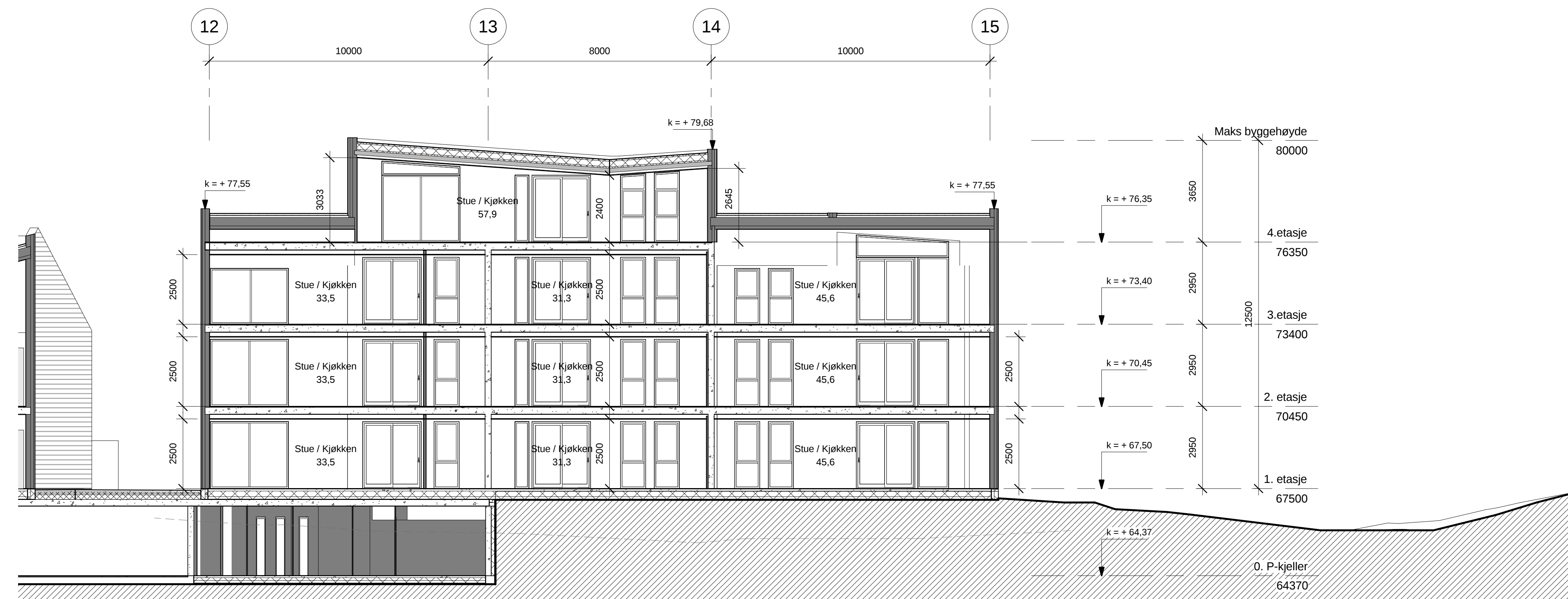
2 Langsnitt Hus C 1 : 100
