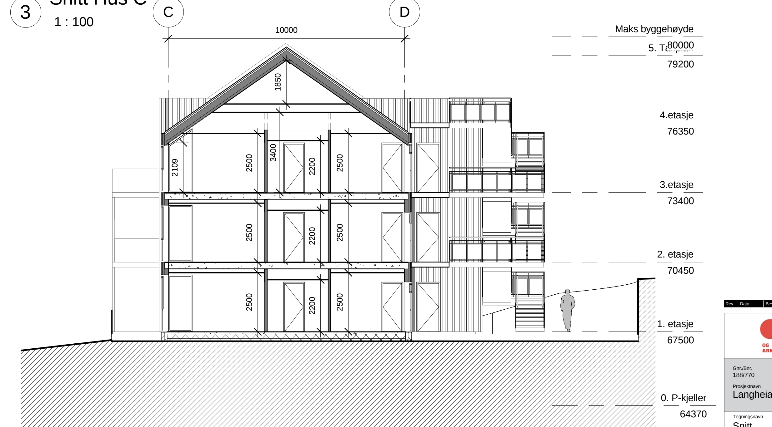
6 Snitt-C04 1 : 100
