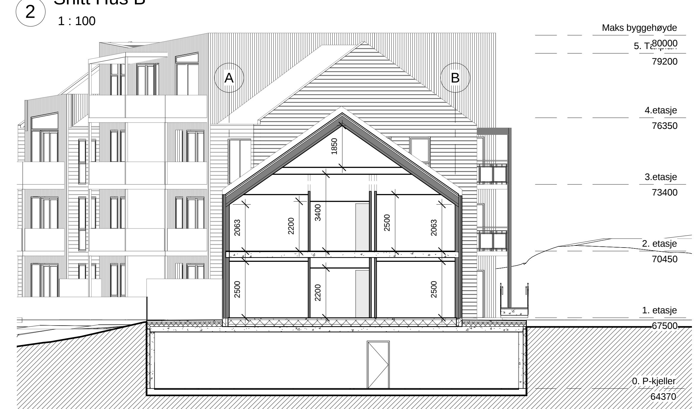
5 Snitt-B04 1 : 100
