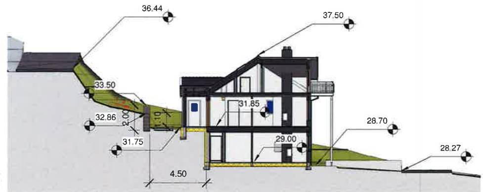
2 Snitt 15 B 1 : 200
