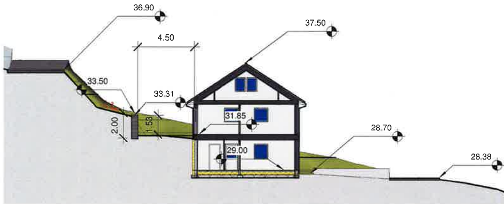
1 Snitt 15 A 1 : 200
