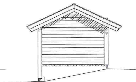
Fasade Nord-vest
