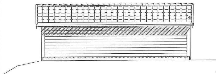
Fasade Nord-Aust
