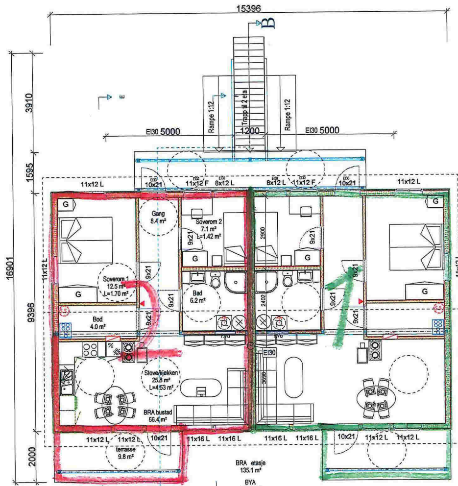
Bustad B BRA 66.5 m2 Alle bustadene lik bustad A SEKSJON 2 Plan 1 eta Bustad A BRA 66.5 m2 SEKSJON 1
