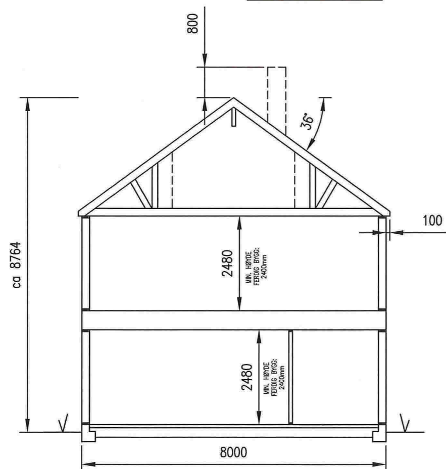
TYPISK SNITT
