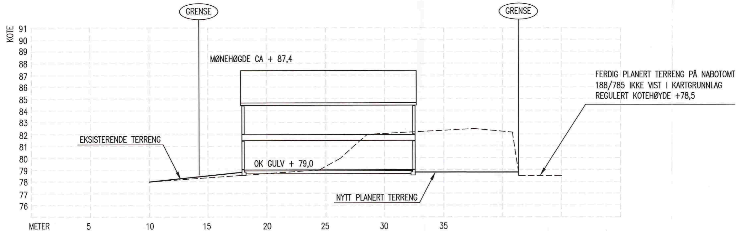
TERRENGSNITT A-A
