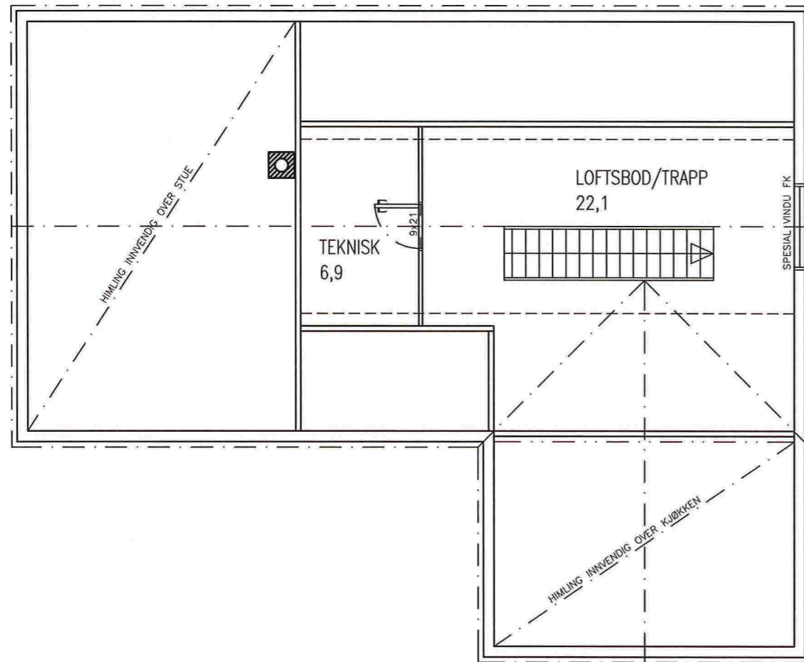
LOFTSPLAN
