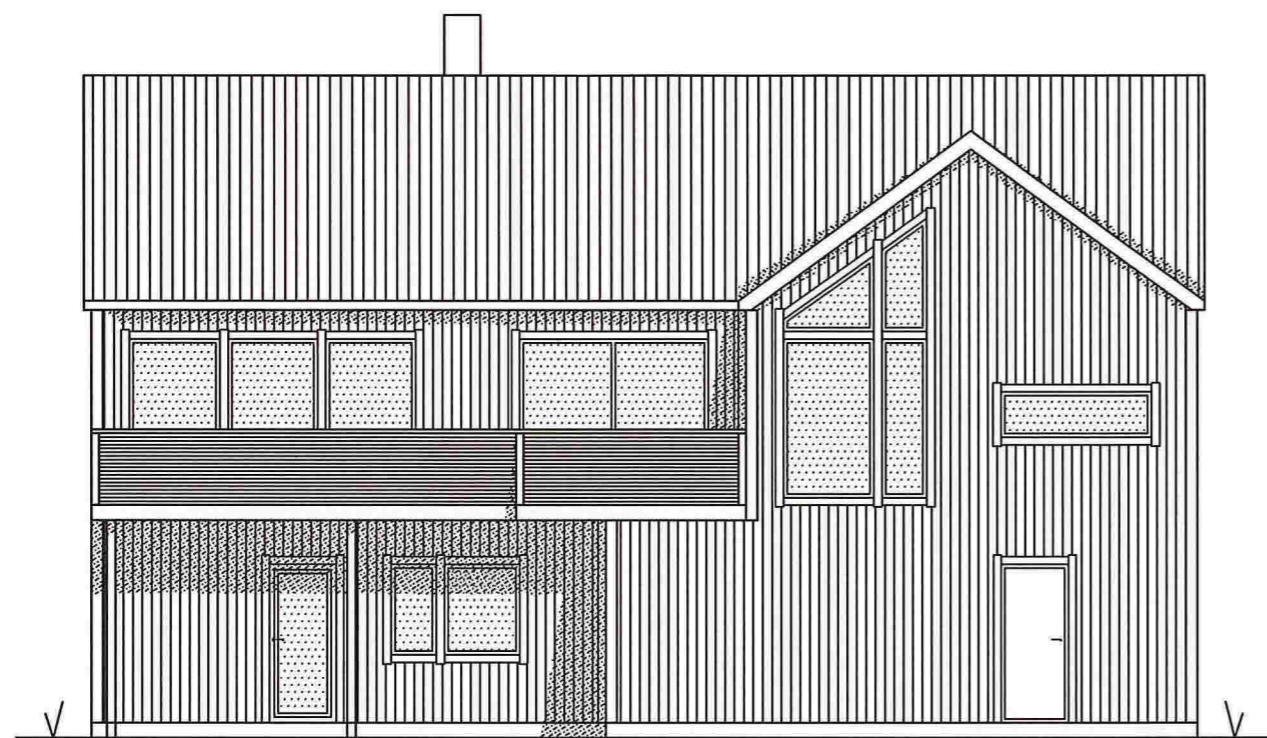
FASADE SØR
