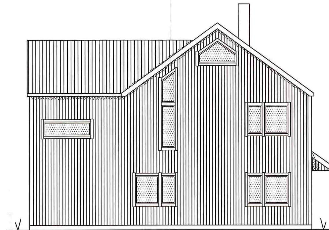
FASADE ØST
