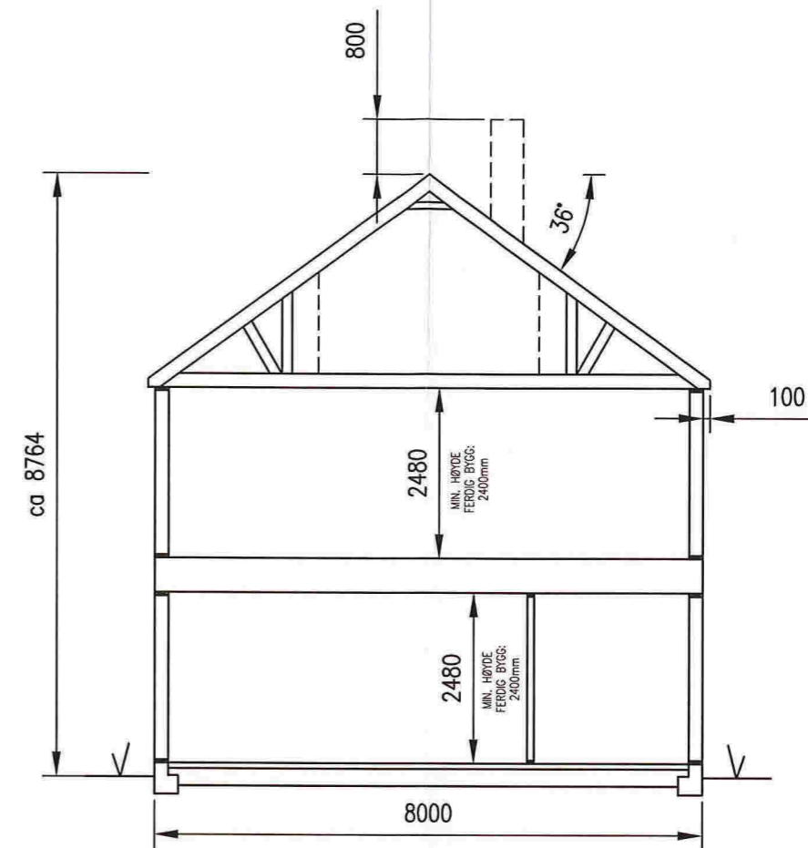
TYPISK SNITT
