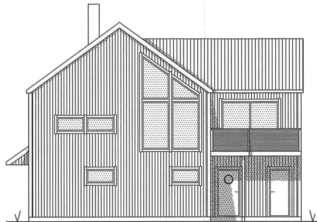
FASADE VEST
