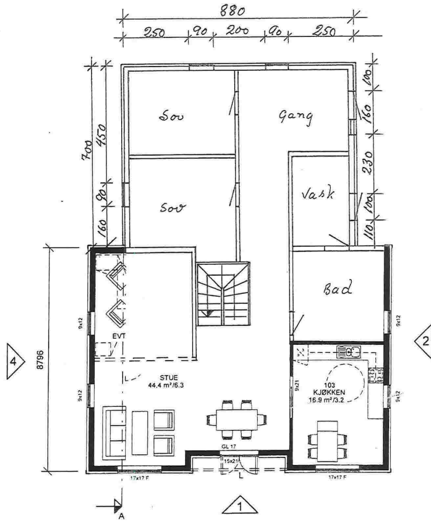
1. ETG.
