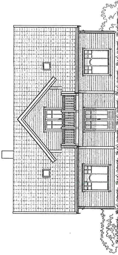
FASADE 1
