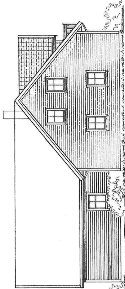
FASADE 4
